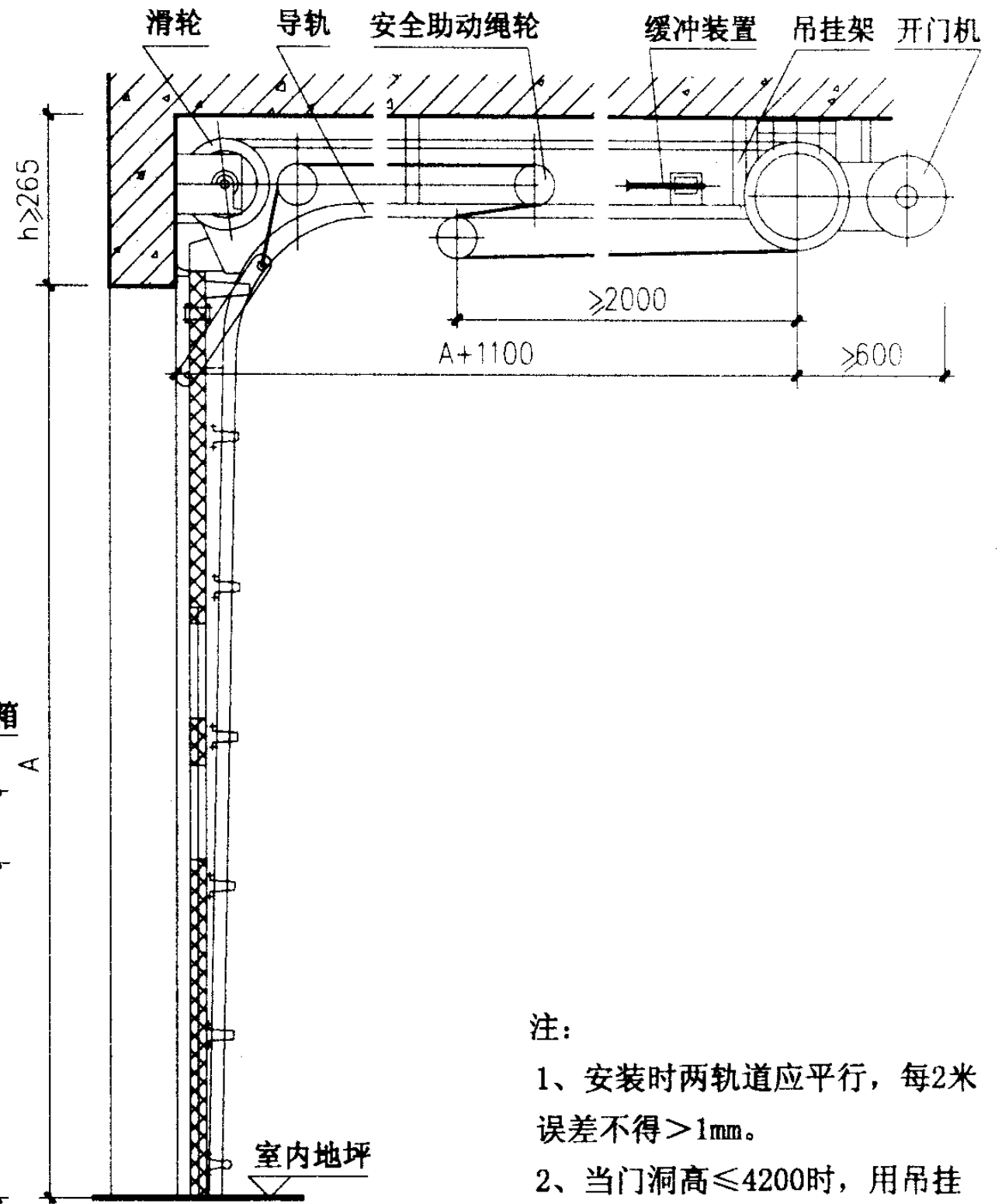
剖面图
