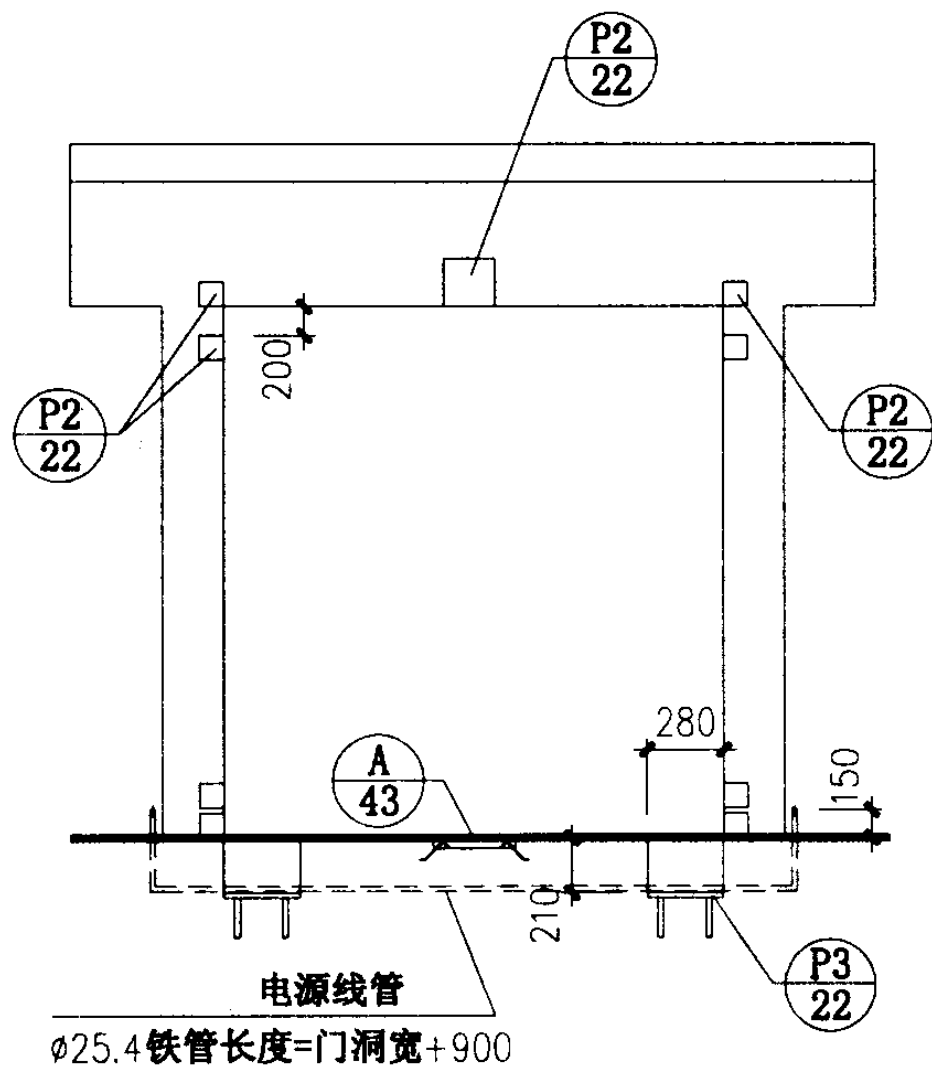
立面图
