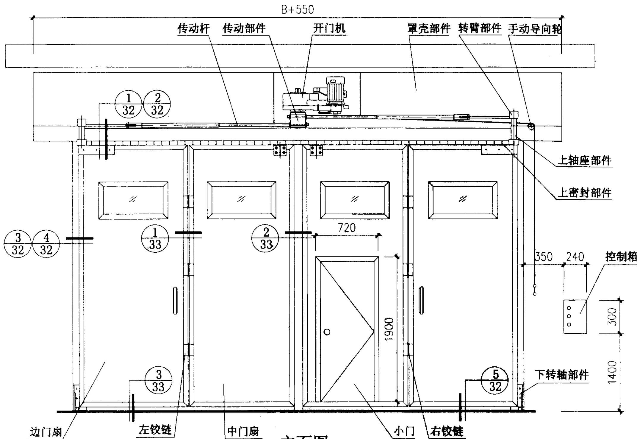
立面图
