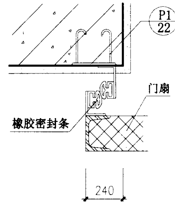
③ 用于混凝土门框
