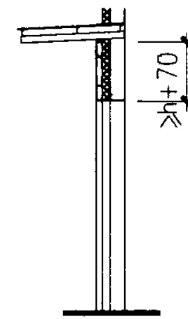
剖面图
