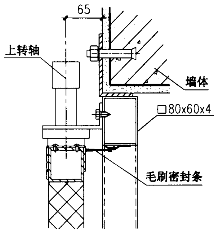
① 用于混凝土门框
