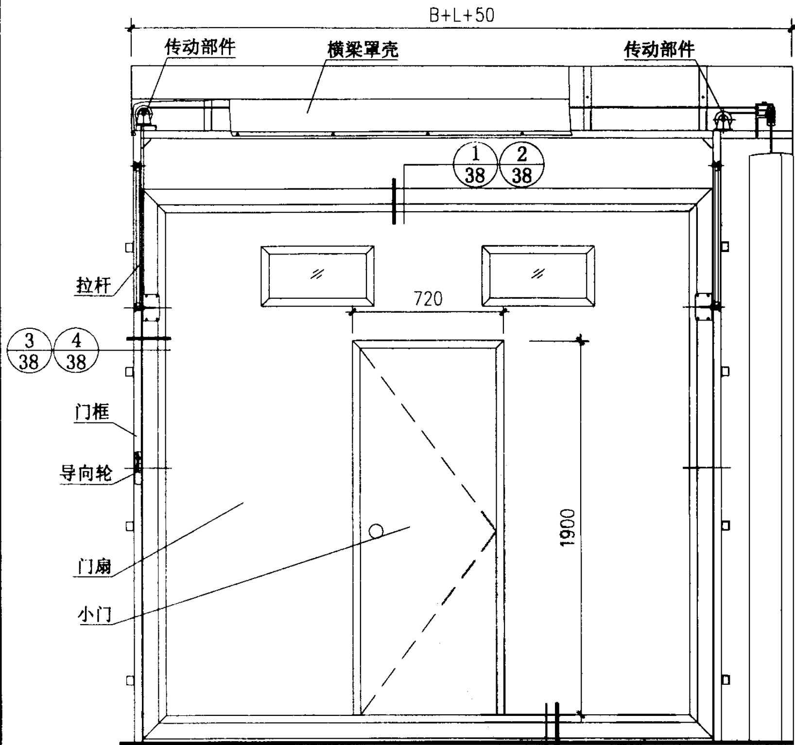
内立面图
