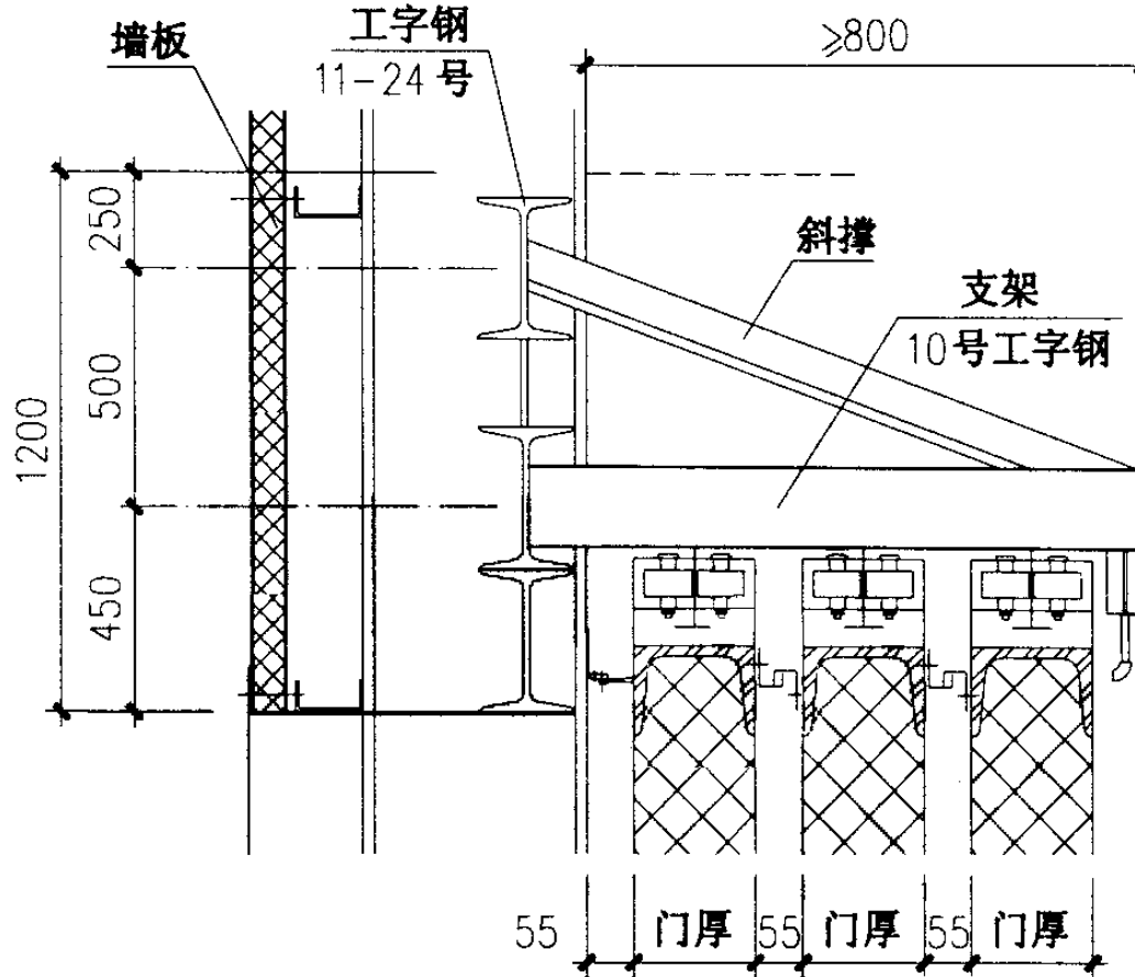
② 用于钢门框
