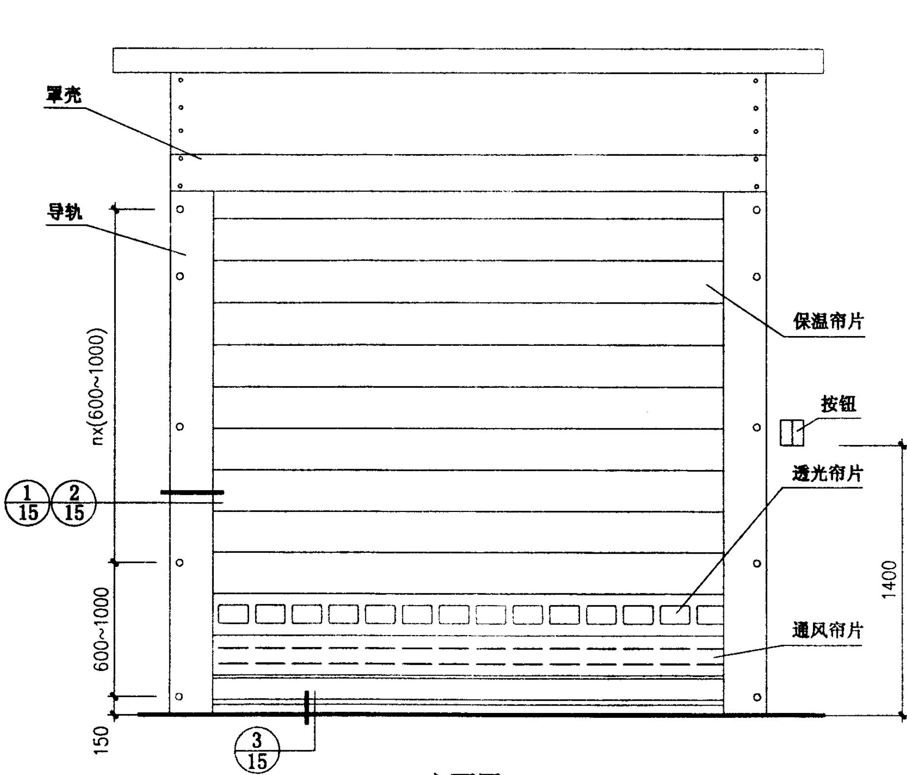
立面图
