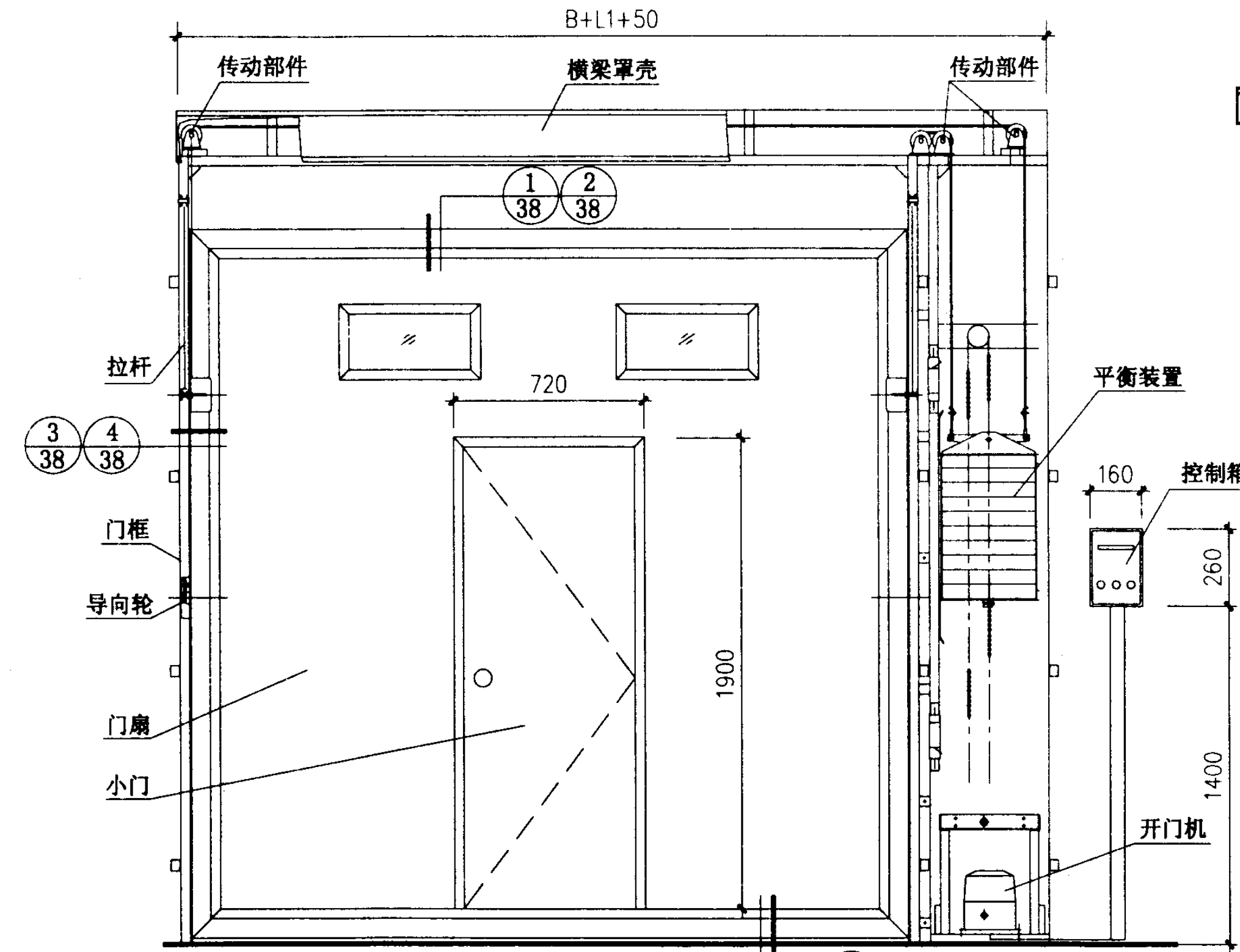
内立面图
