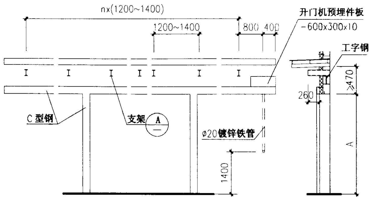
剖面图
