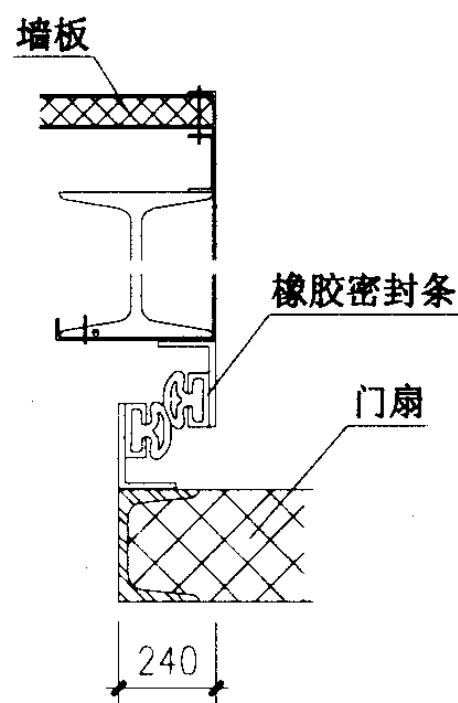
④ 用于钢门框
