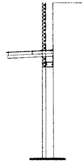
剖面图
