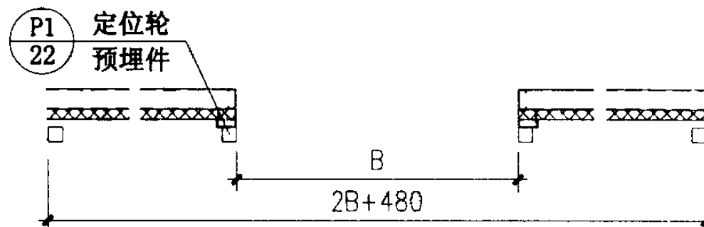
立面图
