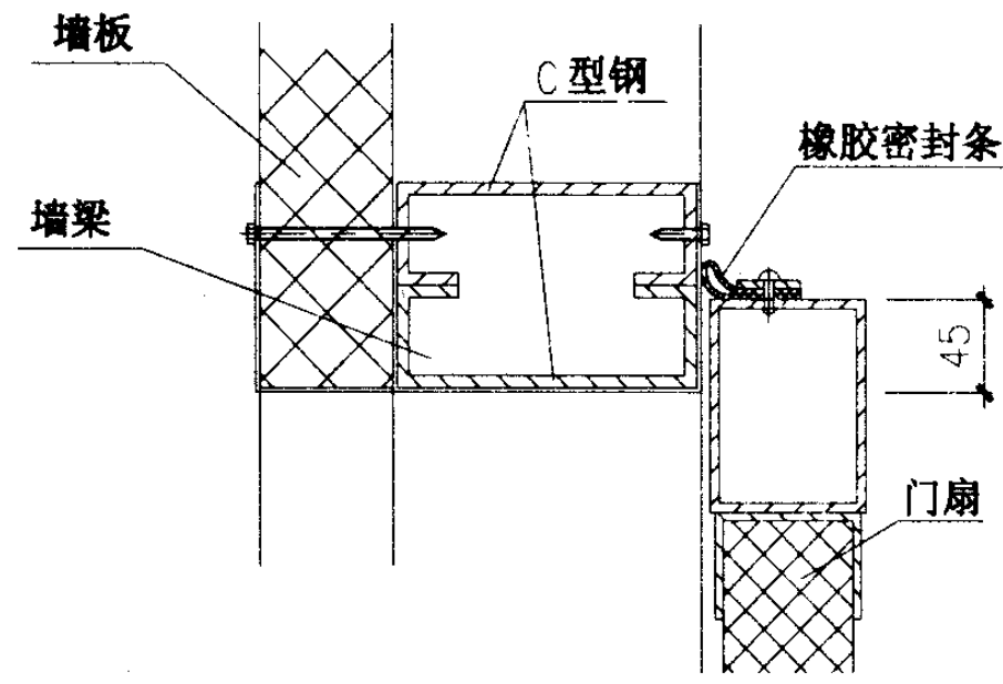
② 用于钢门框
