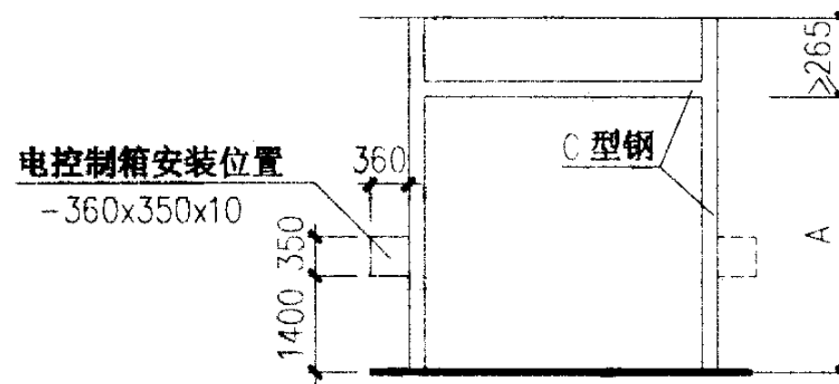
立面图
