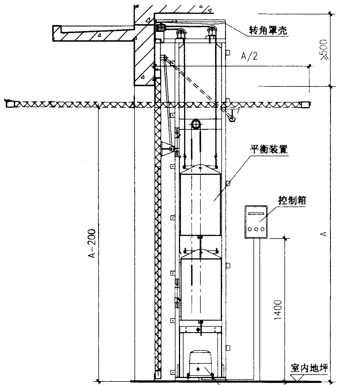
剖面图
