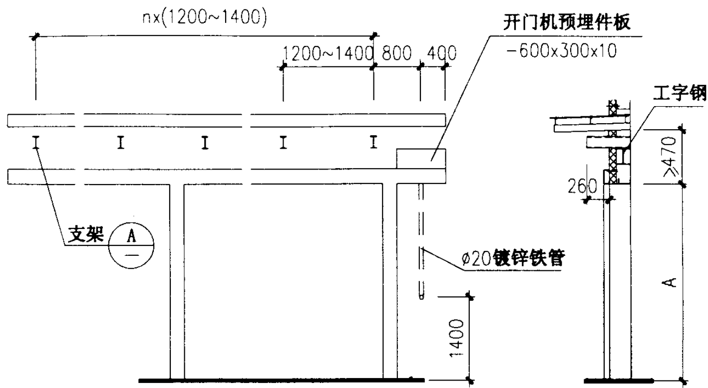
立面图
