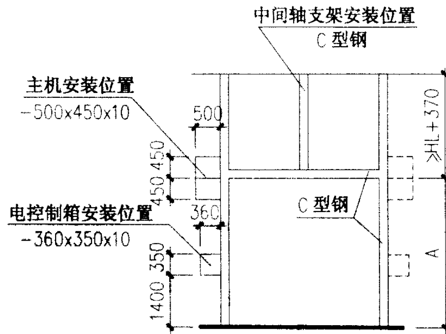
立面图
