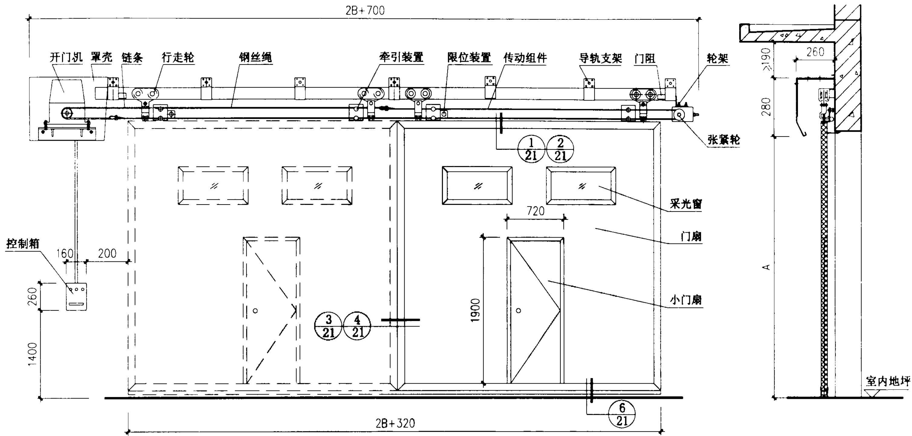
立面图
