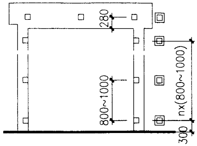
立面图
