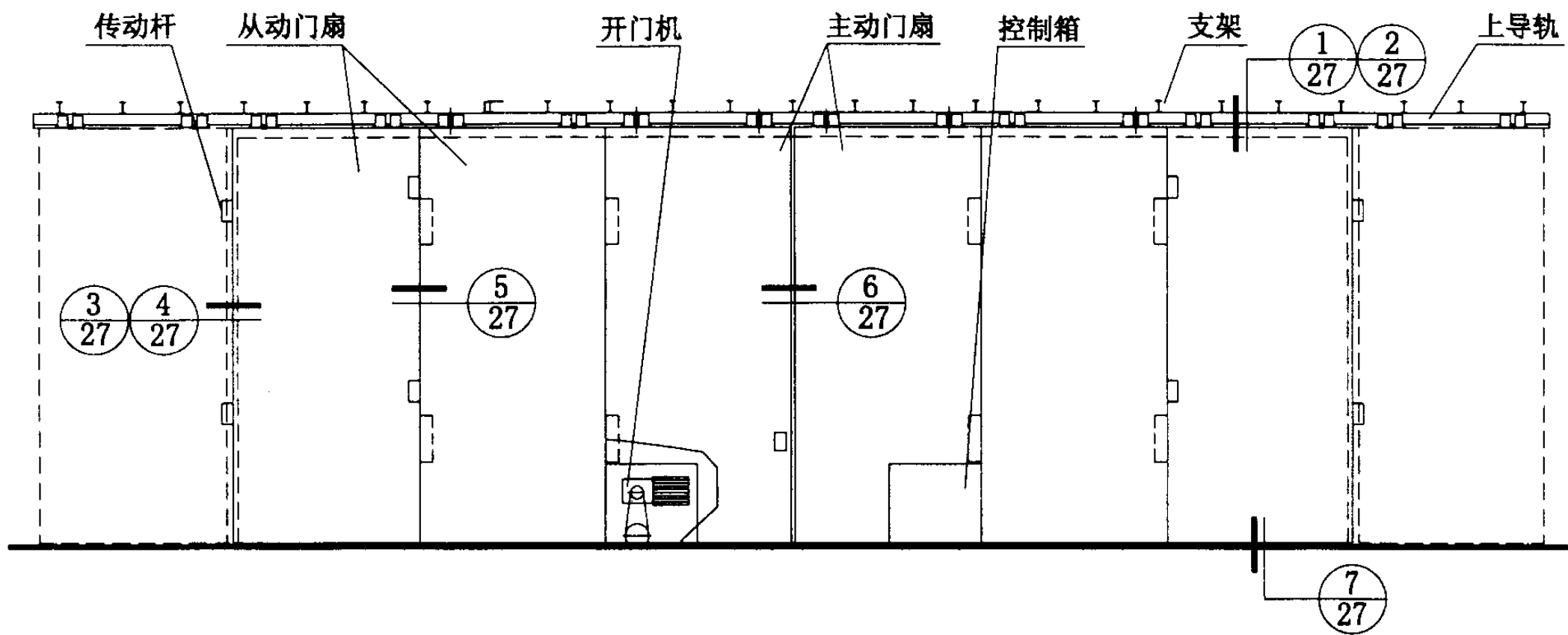
内立面图
