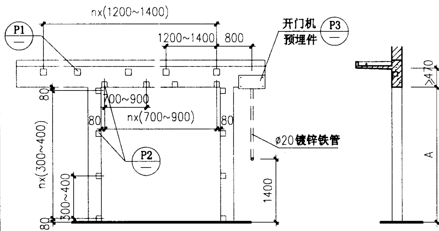
立面图
