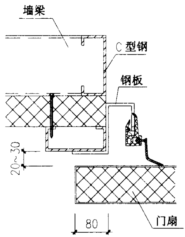
④ 用于钢门框
