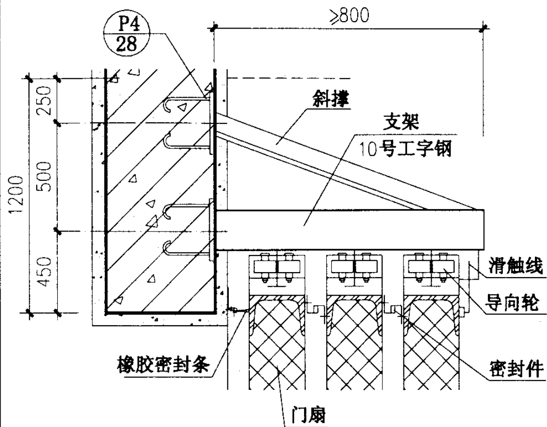
① 用于混凝土门框
