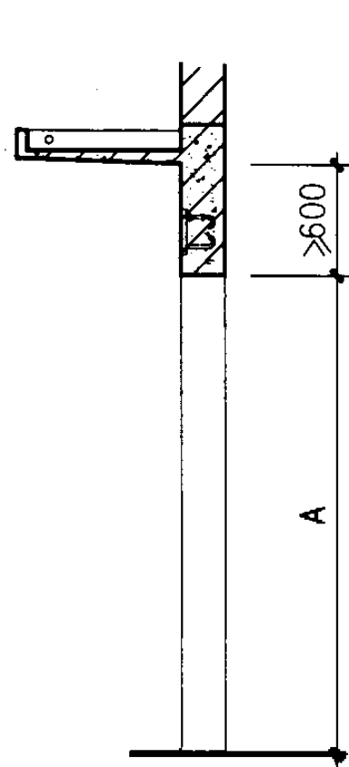
剖面图
