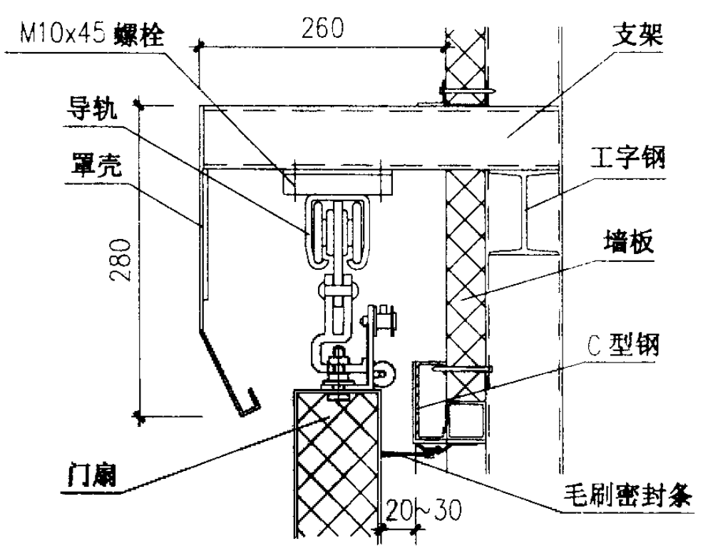
② 用于钢门框
