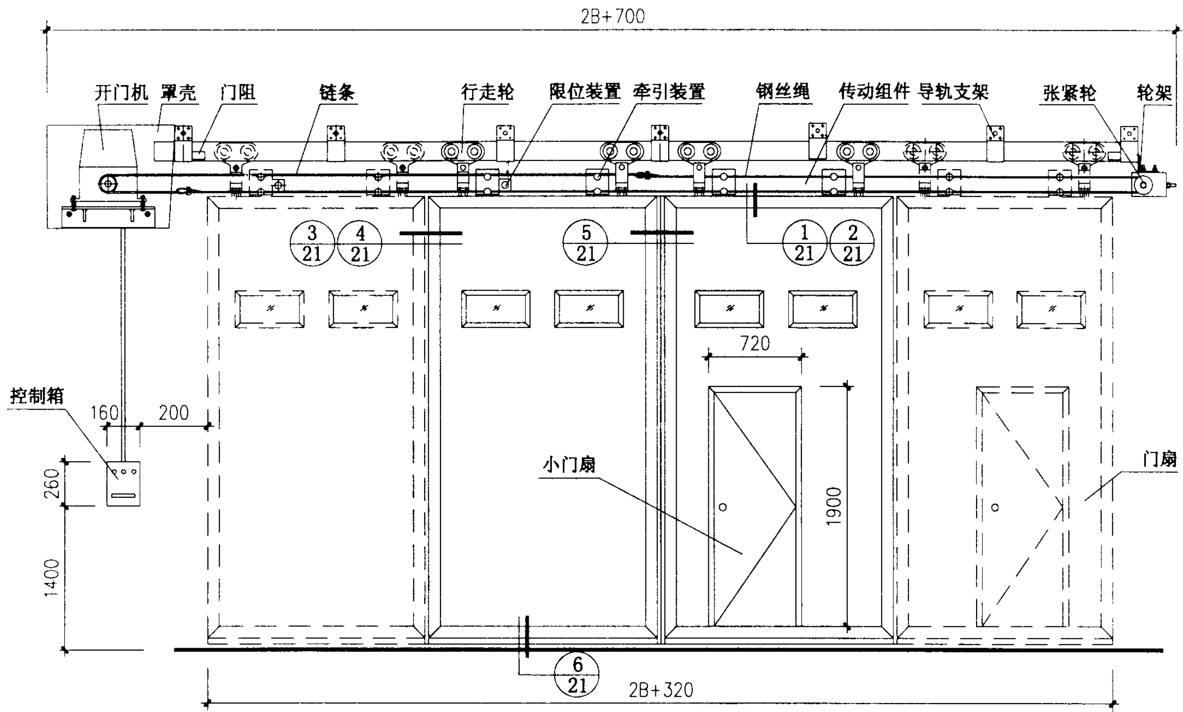
立面图
