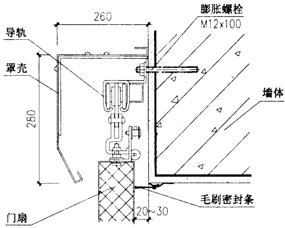
① 用于混凝土门框
