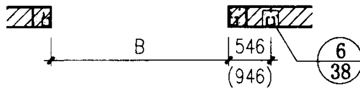
FM1混凝土门框平面图
