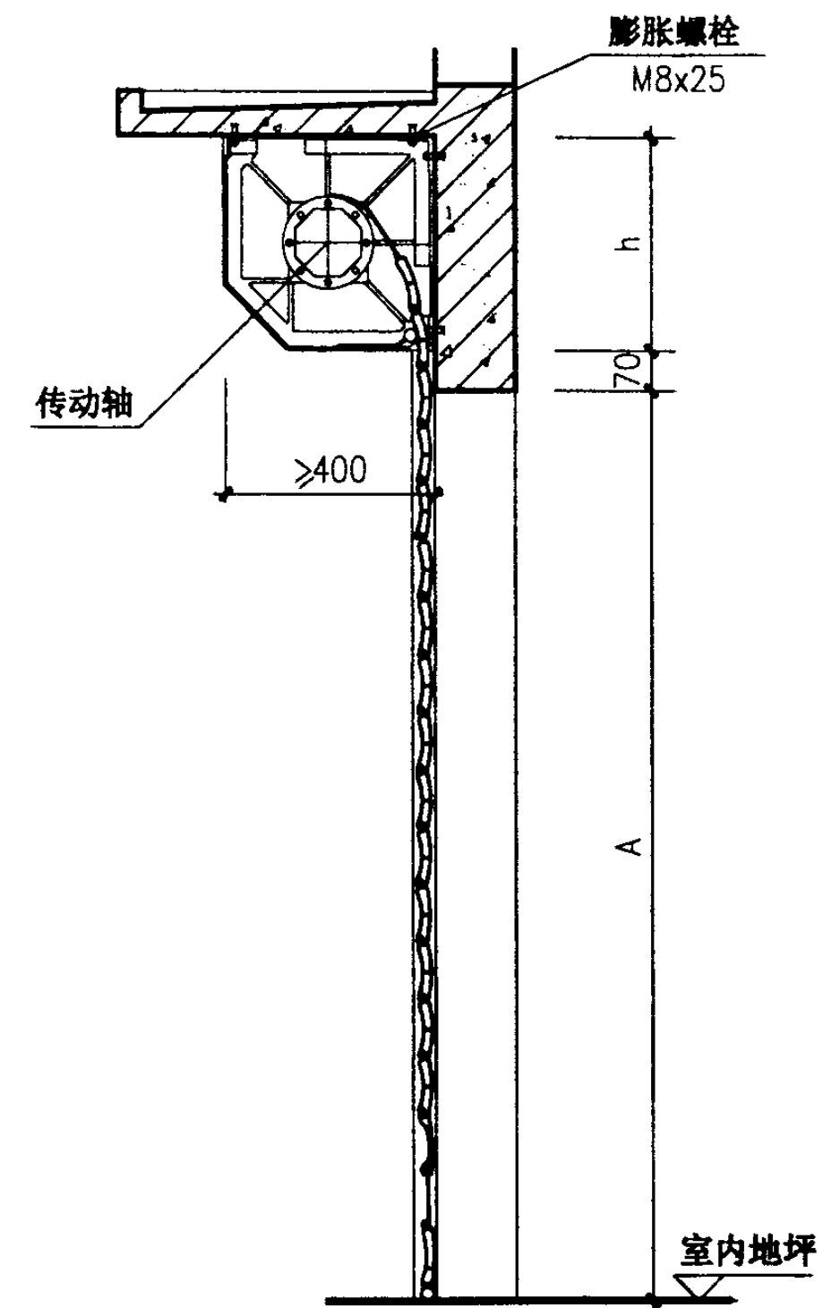
剖面图
