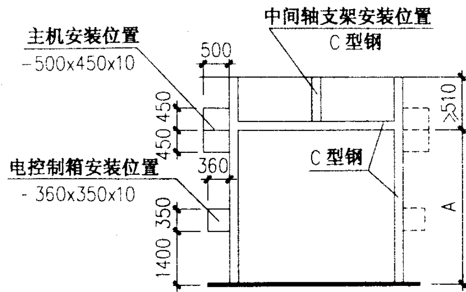
立面图
