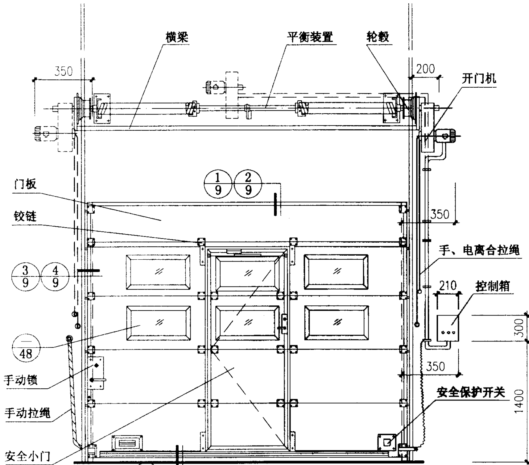
内立面图
