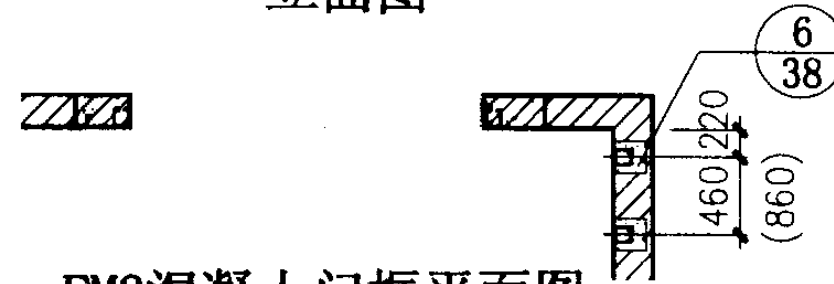
FM2混凝土门框平面图
