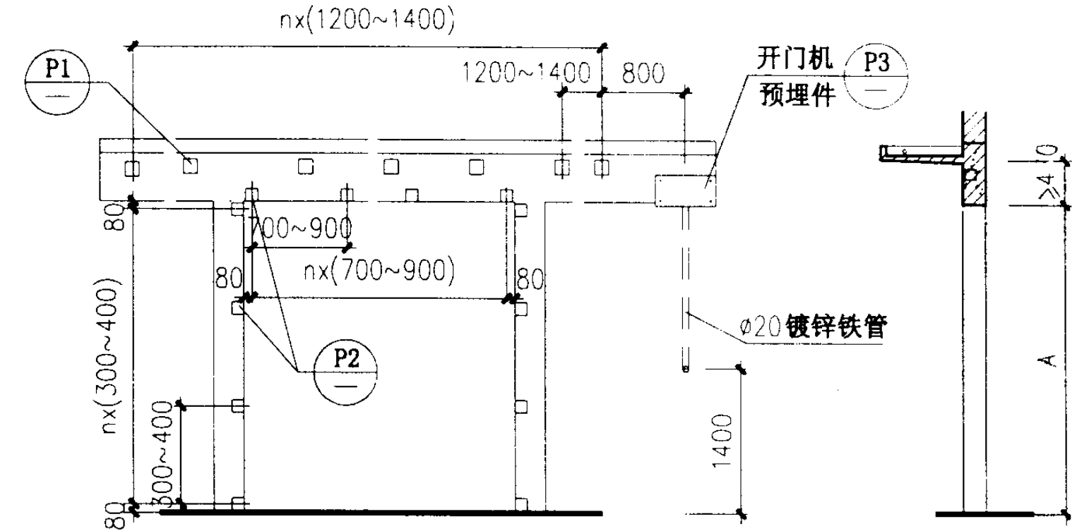
立面图
