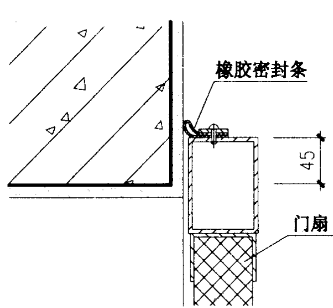
① 用于混凝土门框
