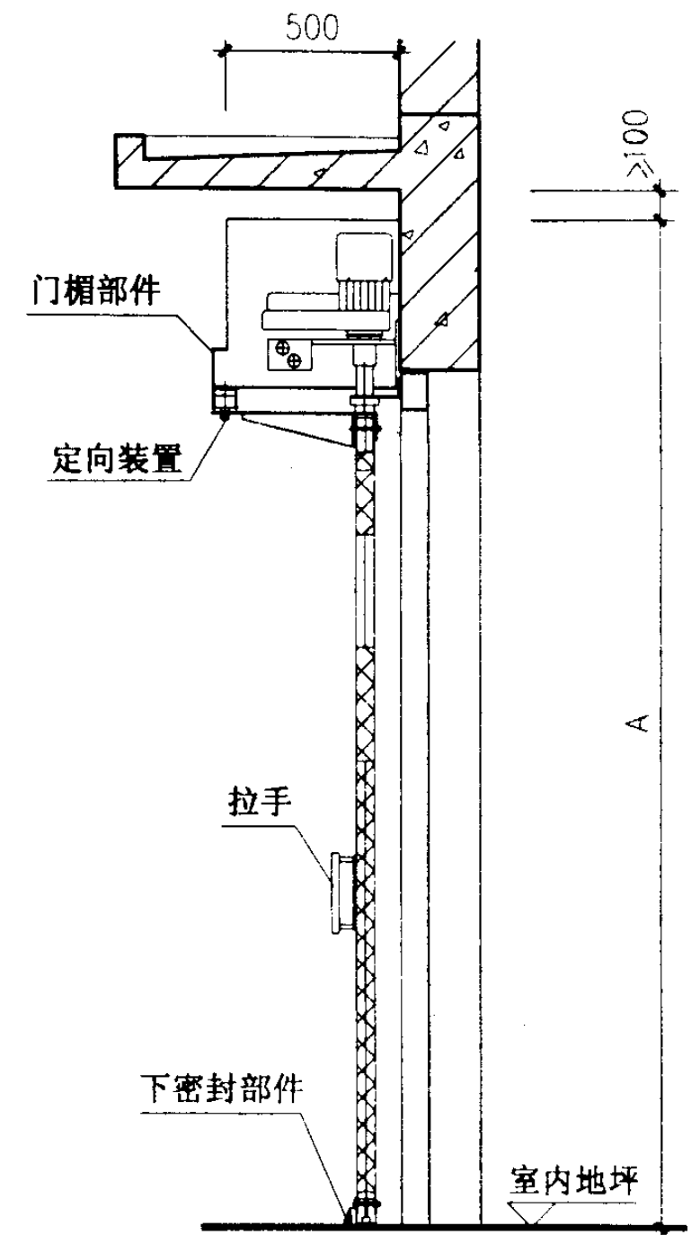
剖面图
