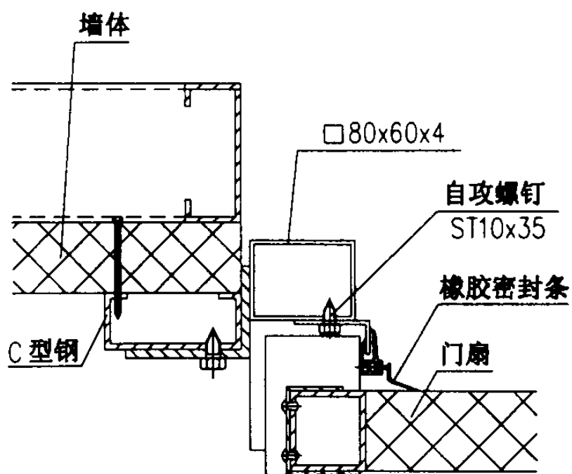
④ 用于钢门框
