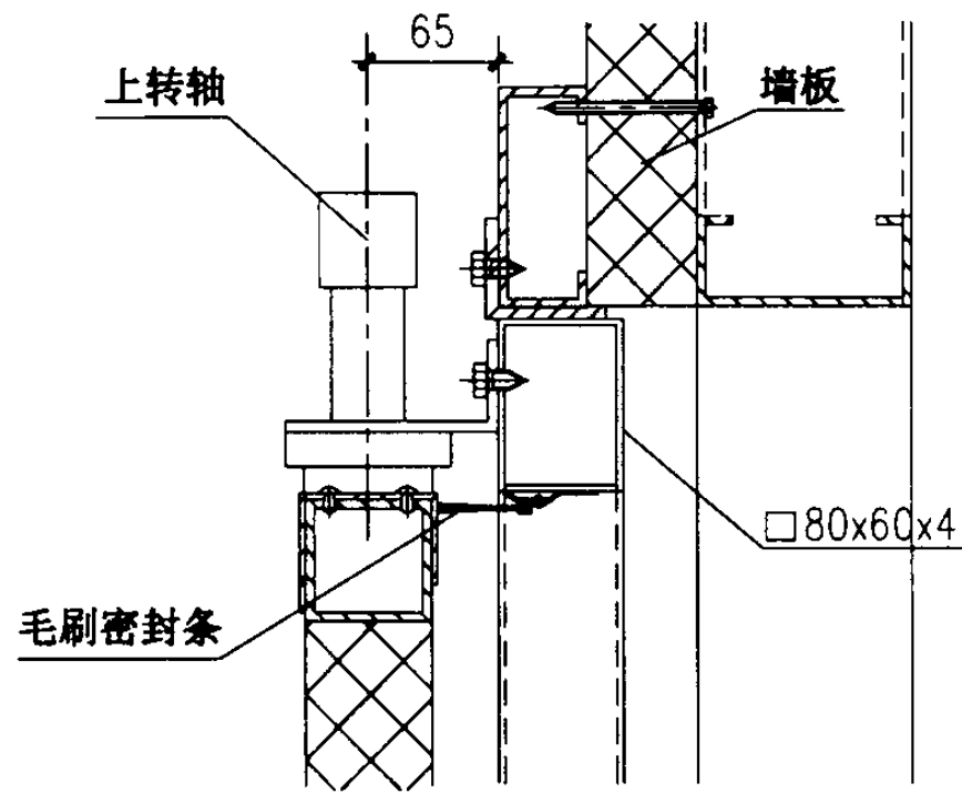
② 用于钢门框
