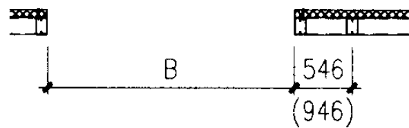
FM1钢门框平面图
