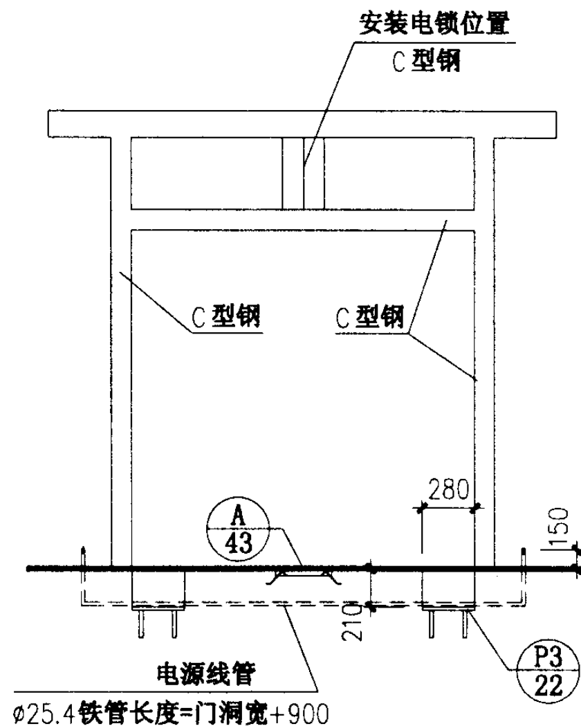
立面图
