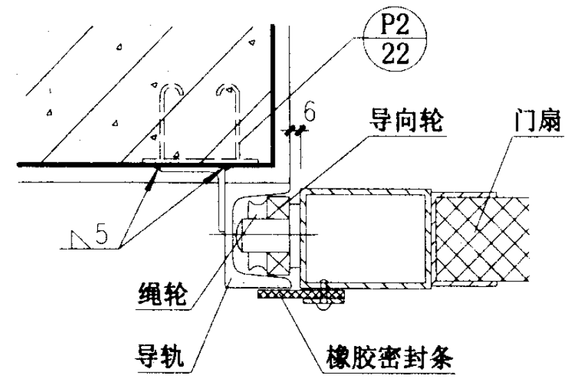
③ 用于混凝土门框
