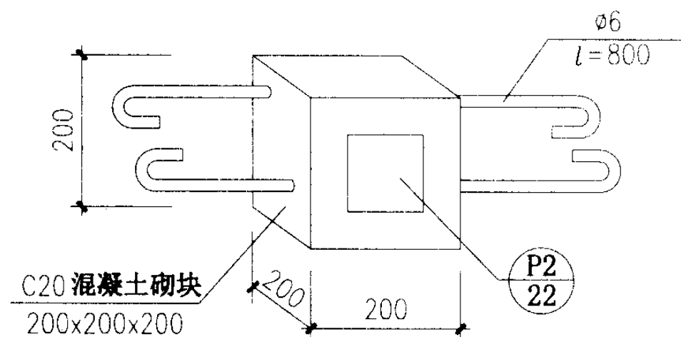
⑥ 混凝土砌块预埋件
