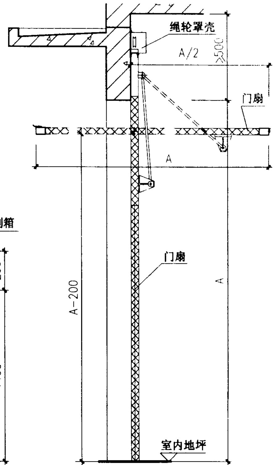
剖面图
