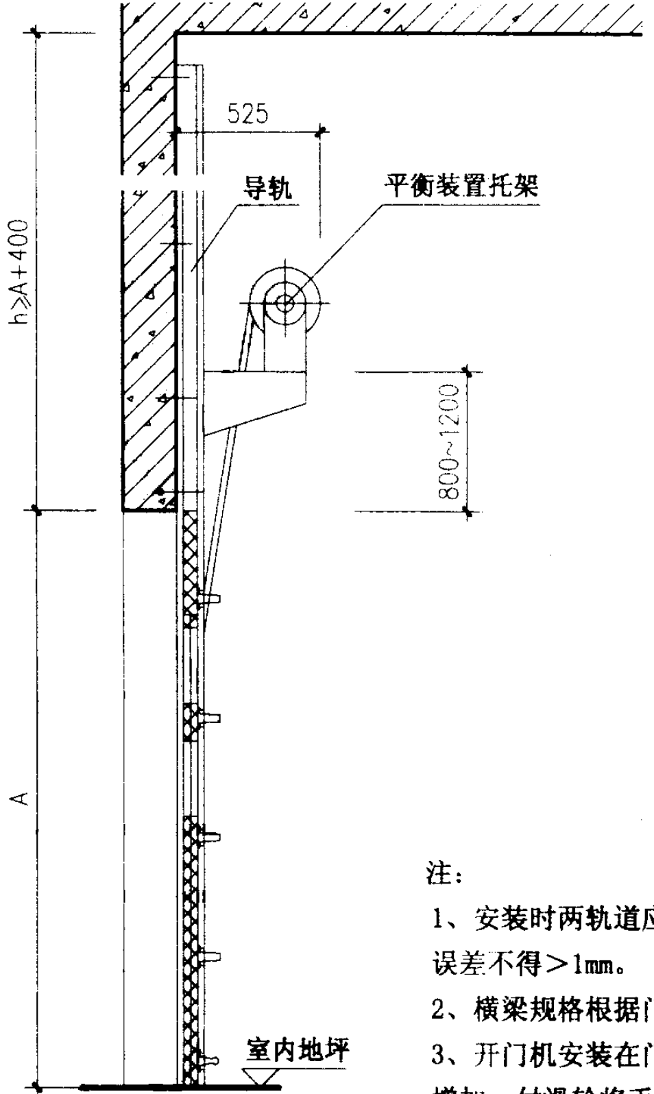
剖面图
