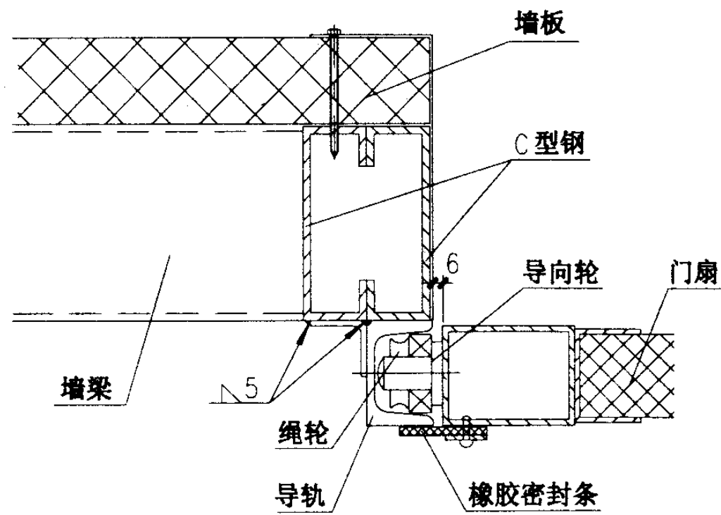
④ 用于钢门框
