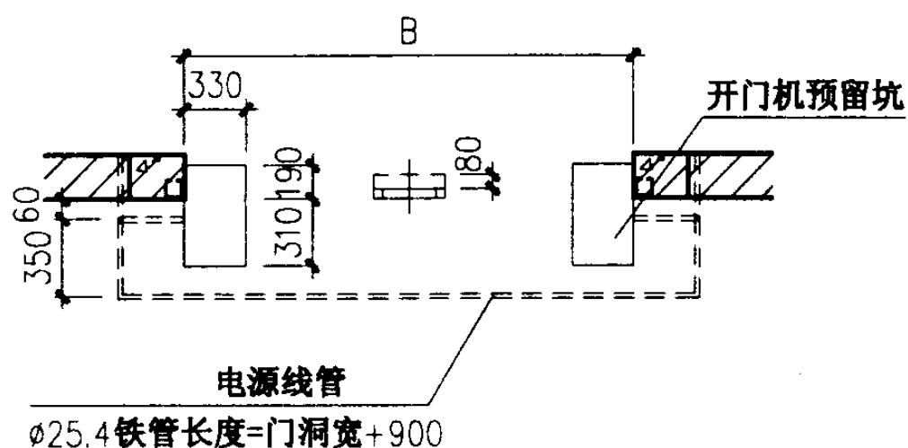
混凝土门框平面图
