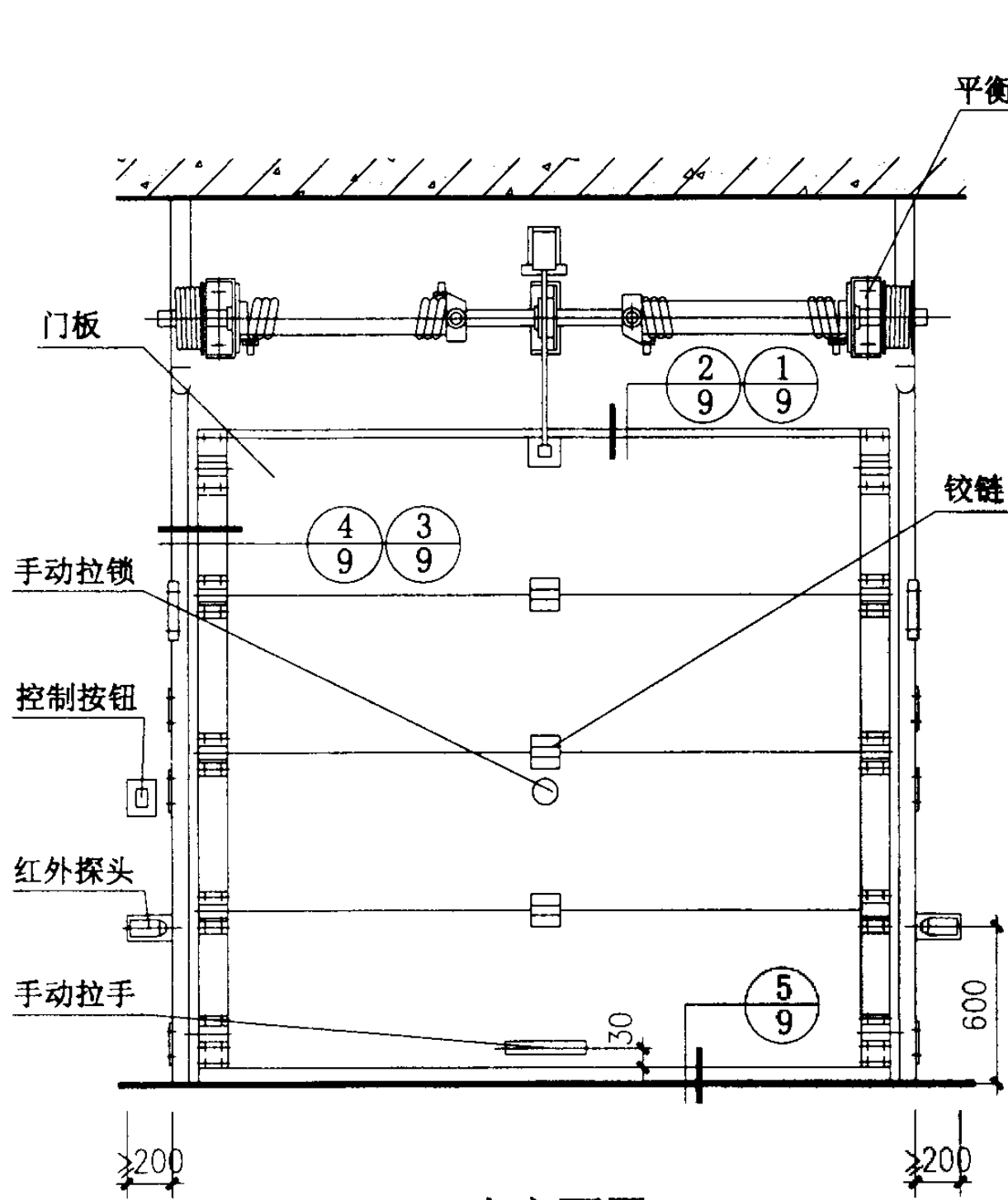
内立面图
