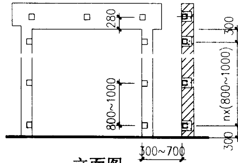
立面图
