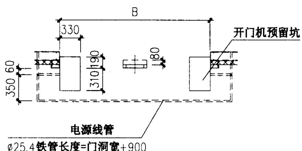
钢门框平面图
