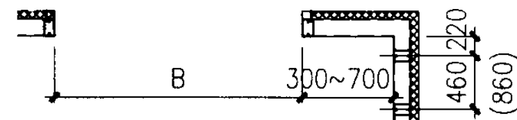
FM2钢门框平面图
