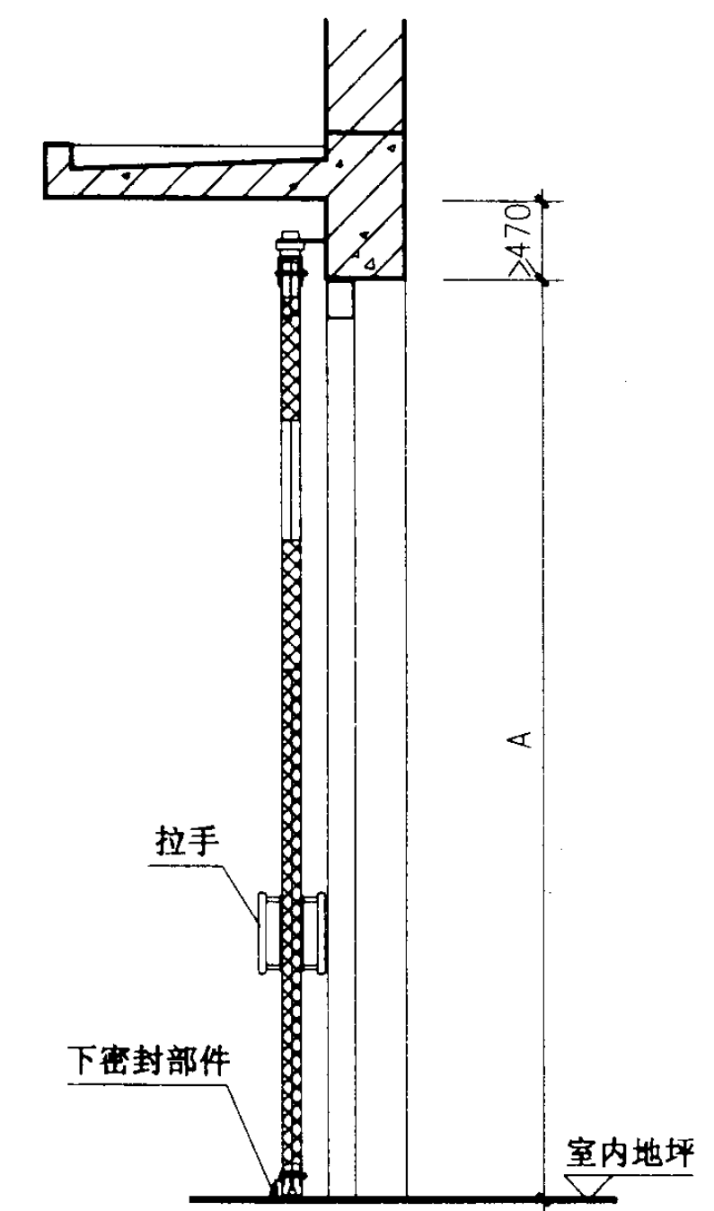
剖面图
