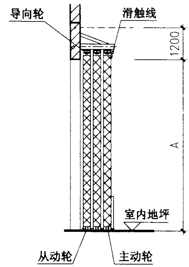
剖面图
