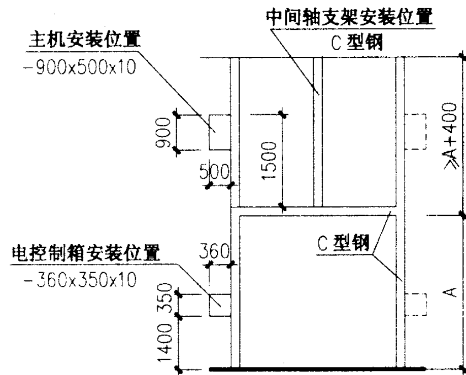
立面图
