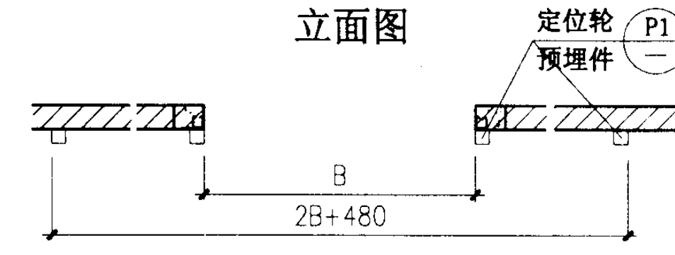
混凝土门框平面图（双向推拉）
