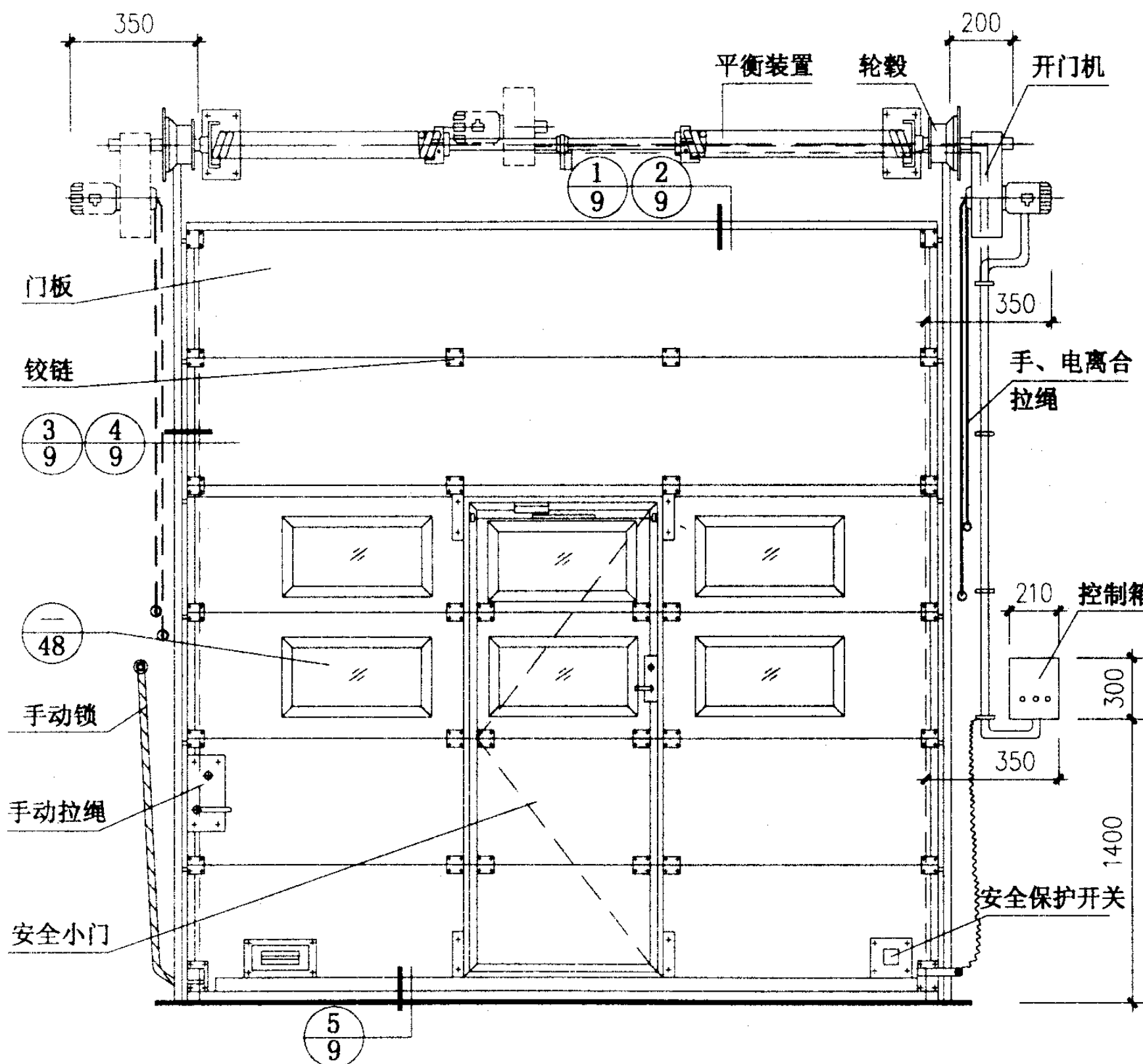
内立面图
