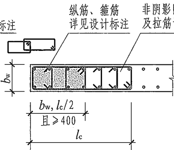
约束边缘暗柱(二) (非阴影区外圈设置封闭箍筋)
