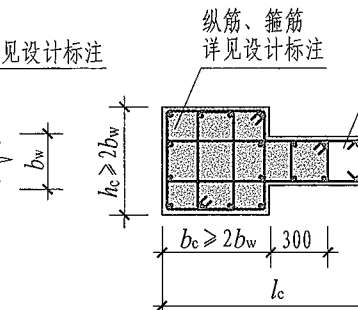
约束边缘端柱(二) (非阴影区外圈设置封闭箍筋)
