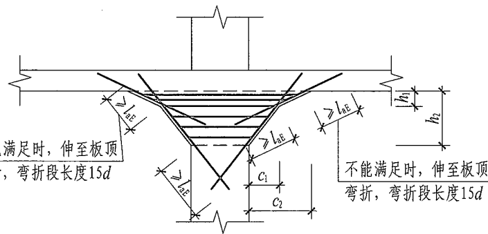
变倾角柱帽ZMc构造
