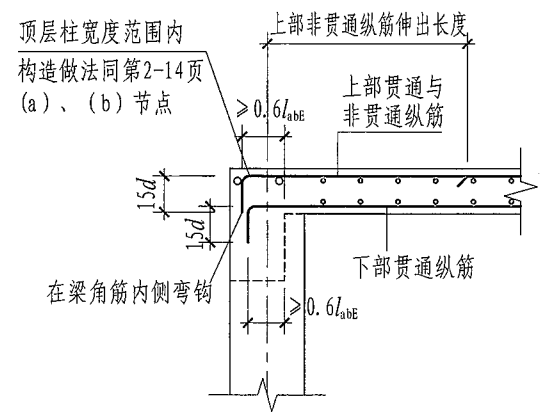
(b) 柱上板带与柱、梁顶层连接
