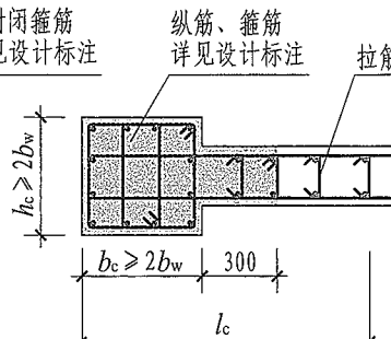
约束边缘端柱(一) (非阴影区设置拉筋)
