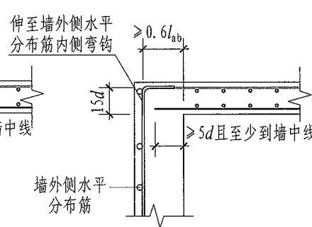
(2) 板端上部纵筋按充分利用钢筋的抗拉强度时
