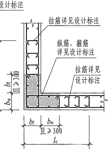
约束边缘转角墙(一) (非阴影区设置拉筋)
