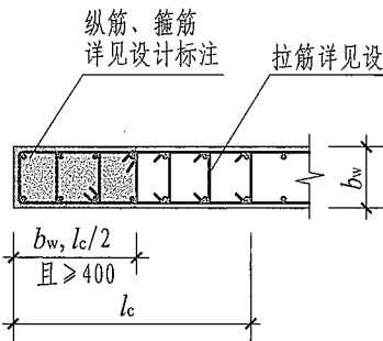
约束边缘暗柱(一) (非阴影区设置拉筋)
