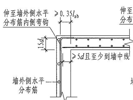
(1) 板端按铰接设计时
