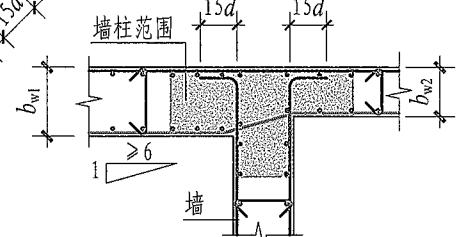
翼墙 (三)
