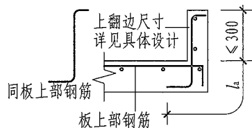
(仅上部配筋)
