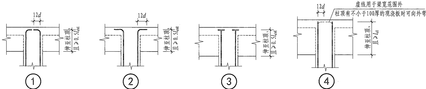
(当柱顶有不小于100厚的现浇板) 柱纵向钢筋端头加锚头(锚板) (当直锚长度 \geq l_{aE} )
