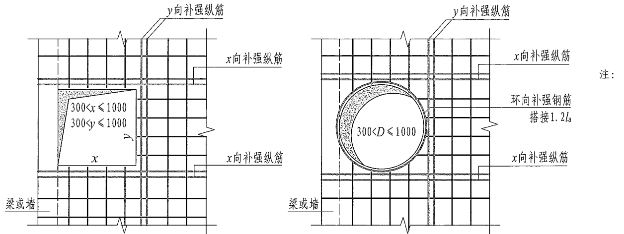
(b) 梁边或墙边开洞
