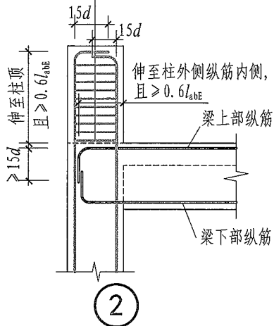
(当伸出长度自梁顶算起不能满足直锚长度 l_{aE} 时)
