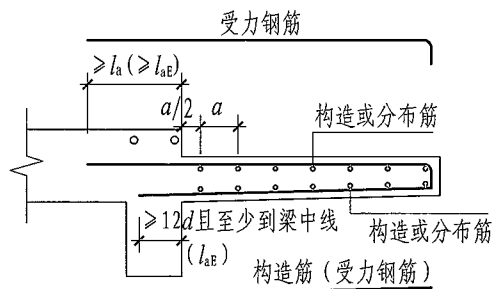
上、下部均配筋
