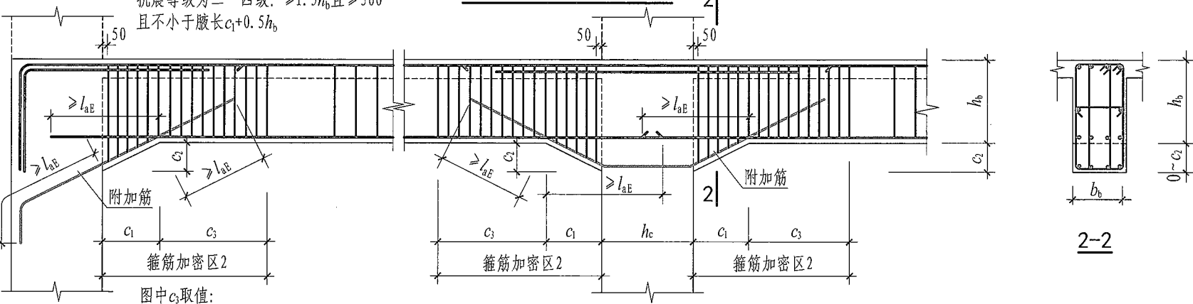
框架梁竖向加腋构造
