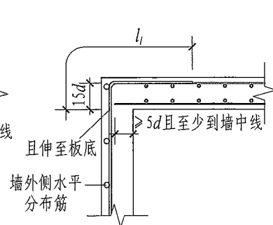
(3) 搭接连接
