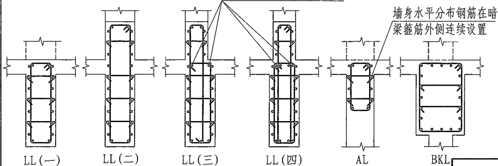
连梁、暗梁和边框梁侧面纵筋和拉筋构造
