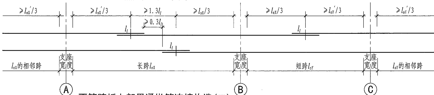
(A) 不等跨板上部贯通纵筋连接构造(一) (B) (C)
