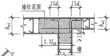
翼墙 (二)
