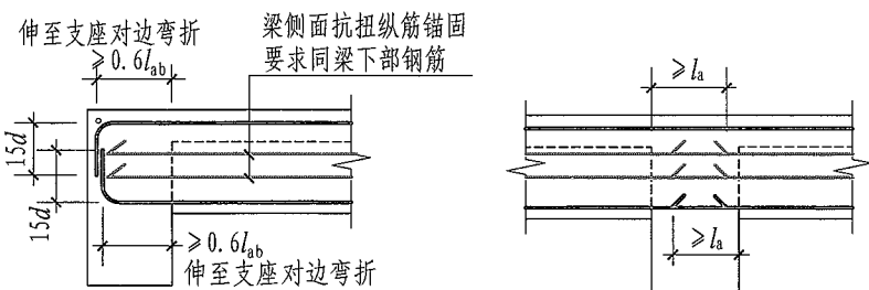
(a) 端支座
