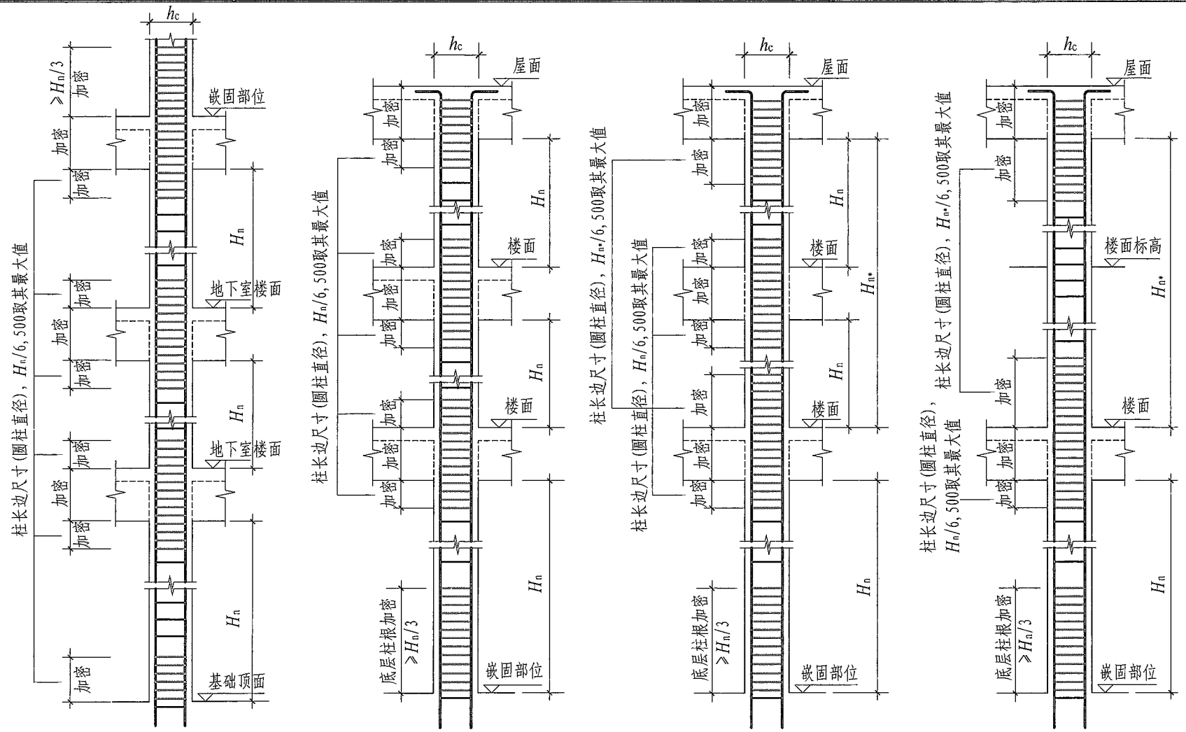
地下室KZ箍筋加密区范围 KZ箍筋加密区范围 单向穿层KZ箍筋加密区范围 双向穿层KZ箍筋加密区范围
