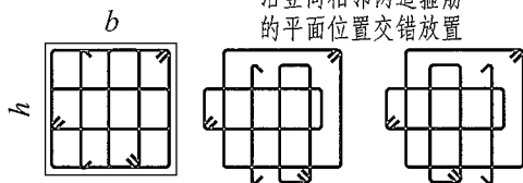
(d) 5×4
