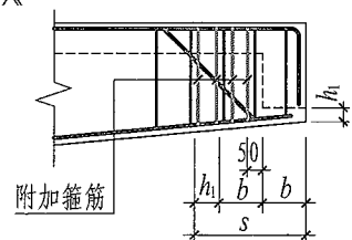
悬挑梁端附加箍筋范围
