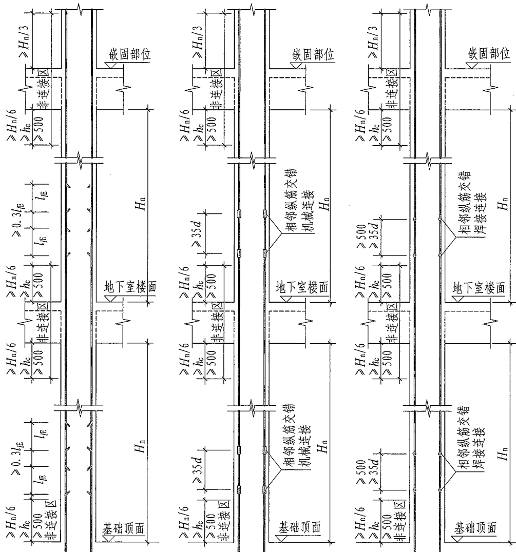
绑扎搭接
