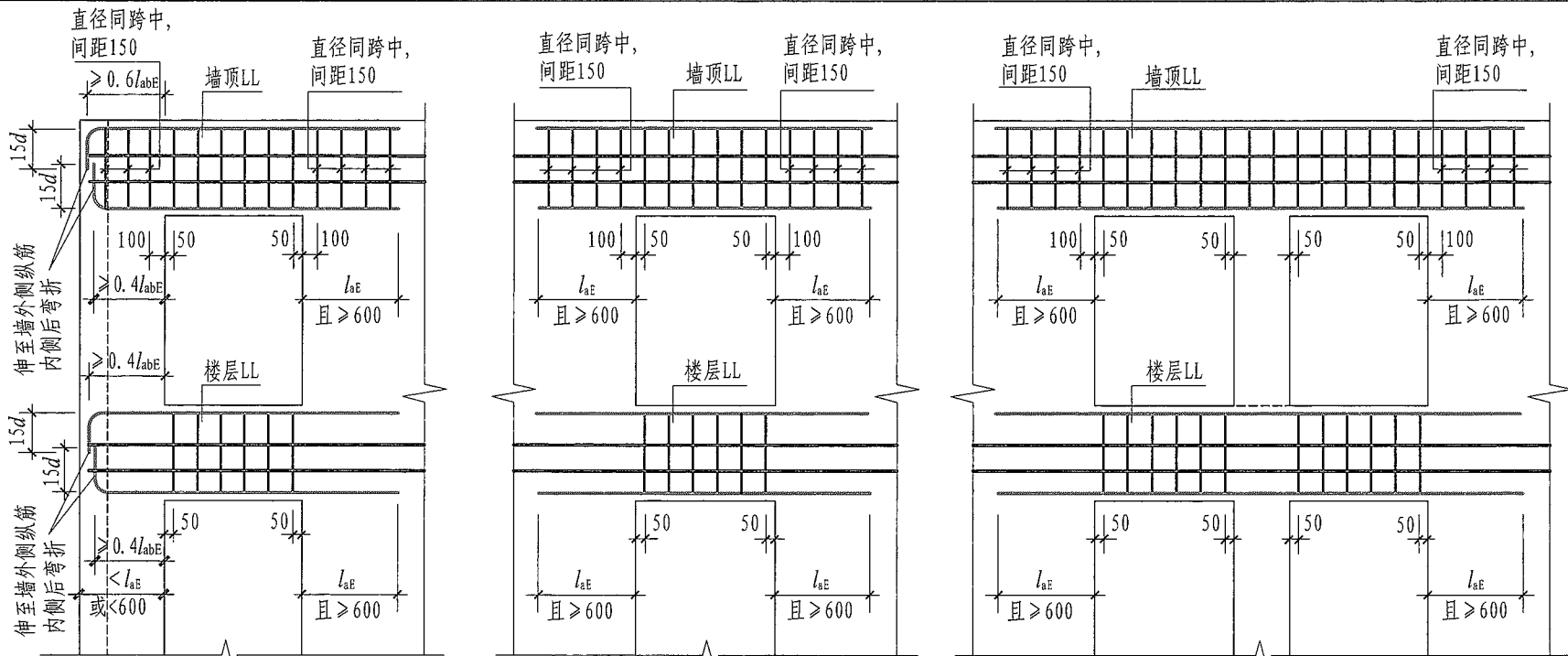
(a) 小墙垛处洞口连梁 (端部墙肢较短)
