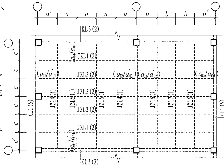
井字梁配筋平面布置图示例
