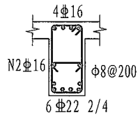
1-1 300 × 550
