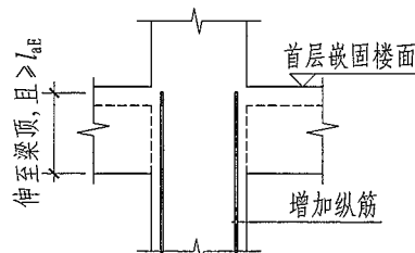
(b) 直锚
