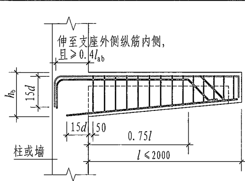
纯悬挑梁XL
