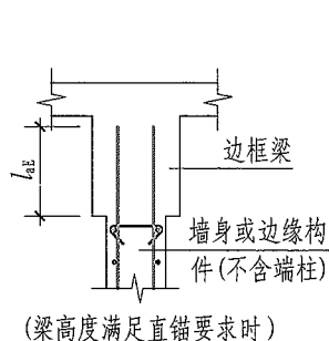
剪力墙竖向钢筋顶部构造
