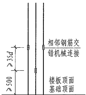
(b) 机械连接
