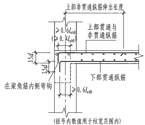
(a) 柱上板带与柱、梁中间层连接
