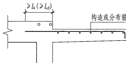
仅上部配筋
