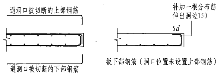
洞边被切断钢筋端部构造
