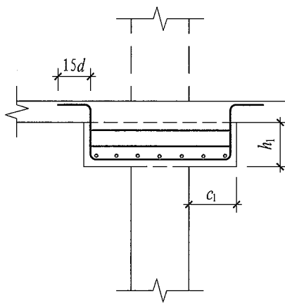
托板柱帽ZMb构造
