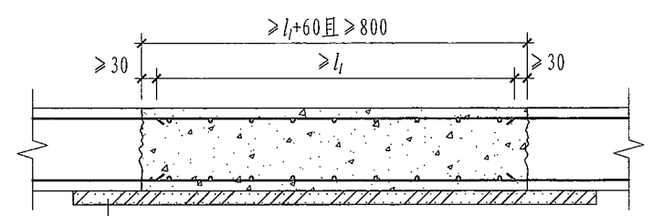
墙后浇带HJD100%搭接钢筋构造
