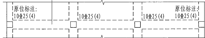
图4.2.5 框架扁梁平面注写方式示例
