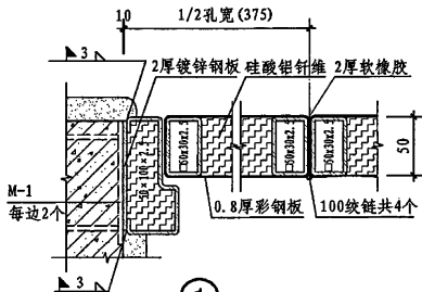
1 人孔盖板详图
