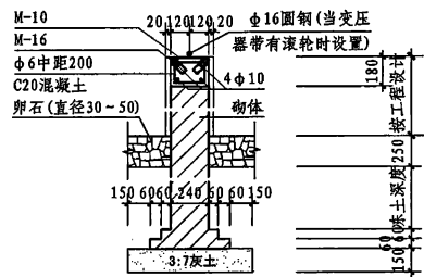
A 墙式变压器基础
