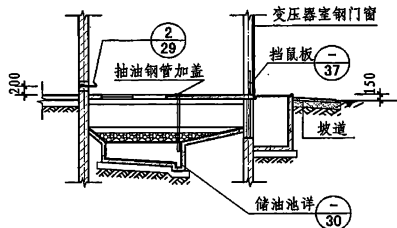
2-2 有风坑式
