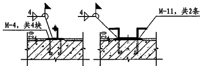
③ 檐口架空引入线拉紧装置埋设件详图
