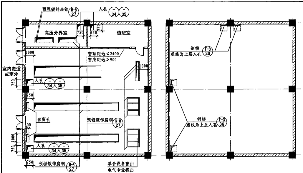
夹层式变电所上层平面图
