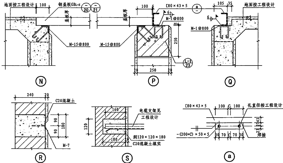
电缆沟节点详图
