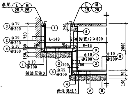
1-1 (钢筋混凝土沟)
