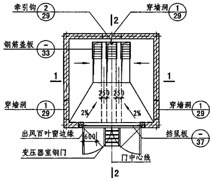
变压器室平面示例
