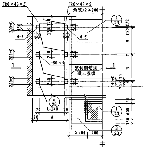
平面 (钢筋混凝土沟壁)
