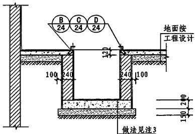
1-1 (砌体沟壁)
