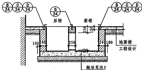
1-1 (砌体沟壁)
