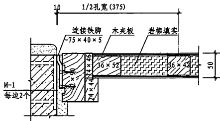
① 人孔盖板详图
