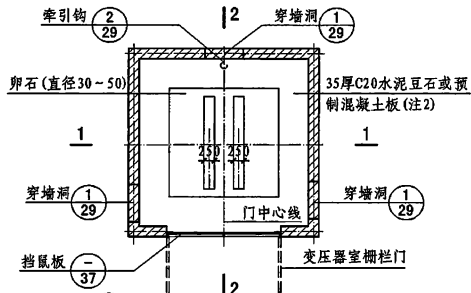
① 敞开低式变压器室平面示例
