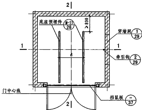
干式变压器室平面示例
