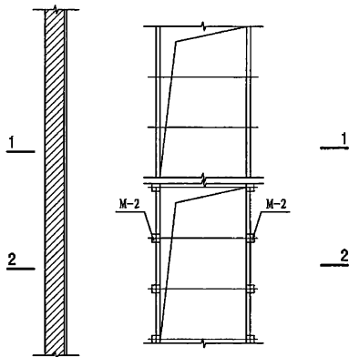
平面 ① (砌体沟壁) ② (混凝土沟壁)
