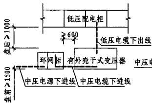
平面电气安全净距示意图1
