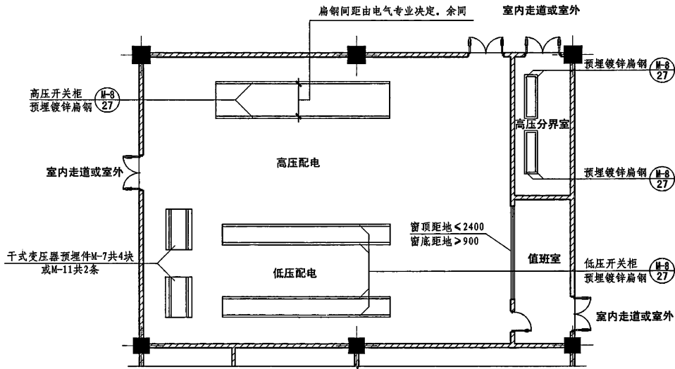
无电缆沟式变配电所平面图
