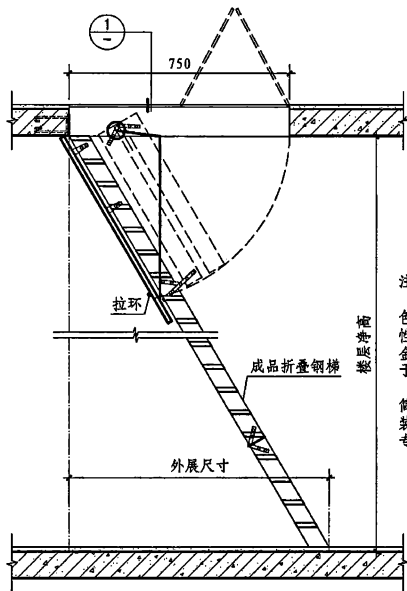
1-1 三截式钢梯展开图
