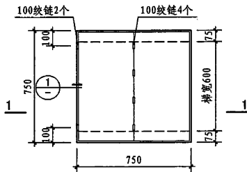
1 检修人孔平面
