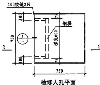
检修人孔详图
