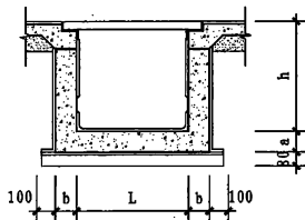
素混凝土电缆沟尺寸示意图
