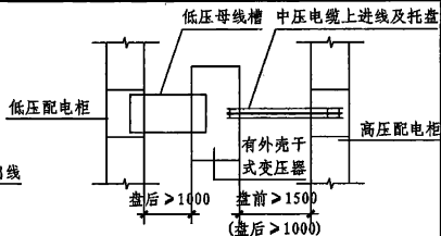
平面电气安全净距示意图3
