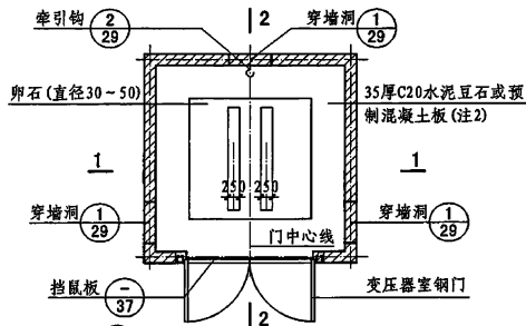
② 封闭低式变压器室平面示例
