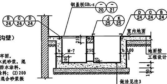
2-2 (混凝土沟壁)
