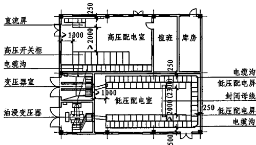
平面电气安全净距示意图2
