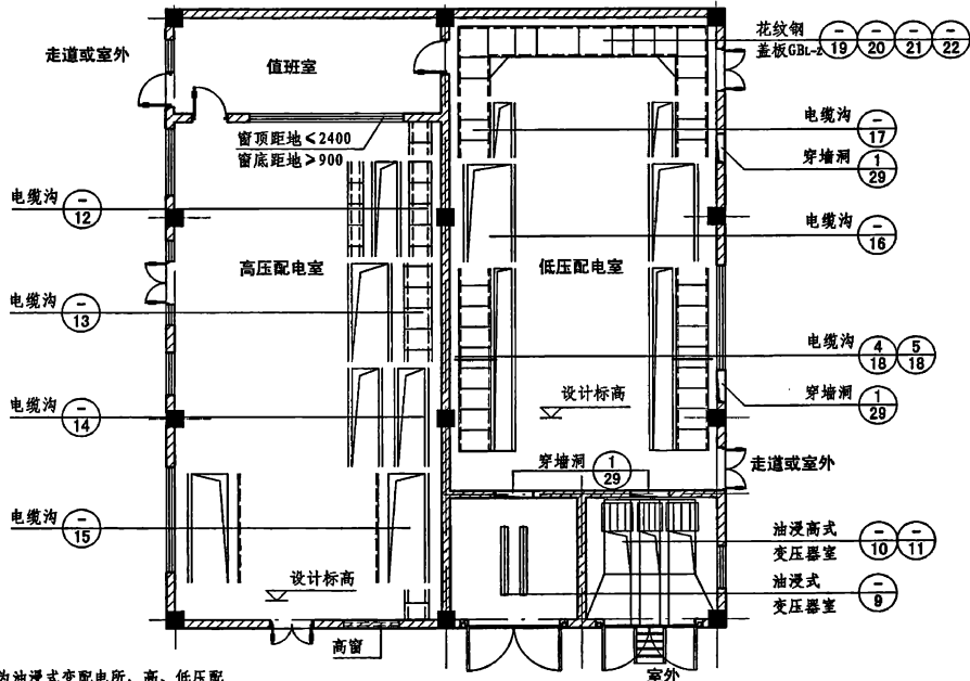
变配电所平面图
