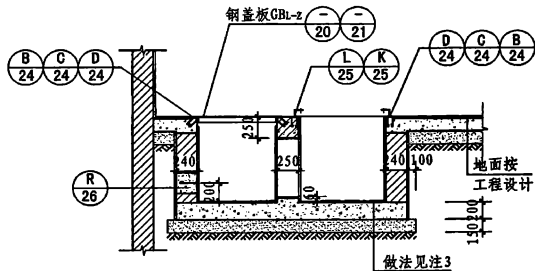
1-1 (砌体地沟)
