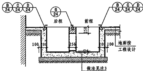
1-1 (混凝土沟壁)
