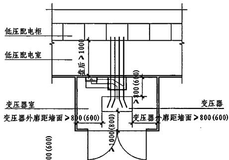
平面电气安全净距示意图1
