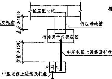
平面电气安全净距示意图5
