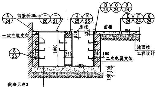
1-1 (砌体沟壁)
