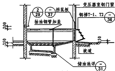
2-2 无风坑式
