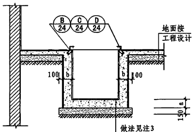
2-2 (混凝土沟壁)
