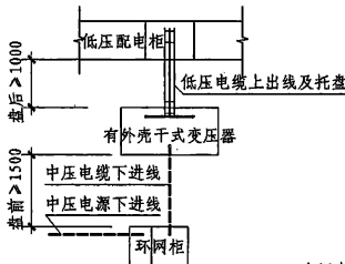
平面电气安全净距示意图4
