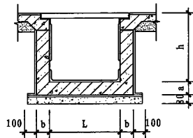
钢筋混凝土电缆沟尺寸示意图
