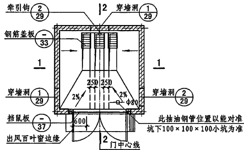
变压器室平面示例
