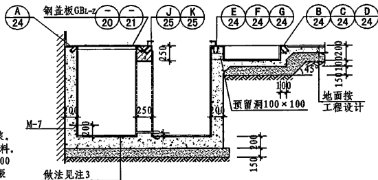
1-1 (混凝土沟壁)
