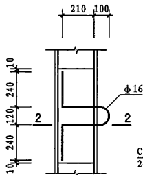
② 牵引钩平面
