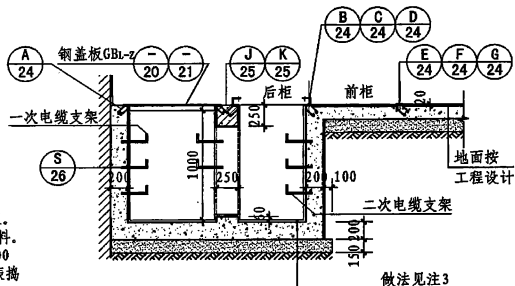
1-1 (混凝土沟壁)
