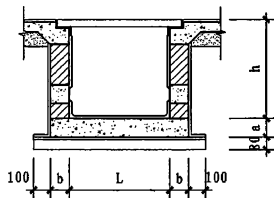
砌体电缆沟尺寸示意图
