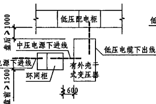
平面电气安全净距示意图2
