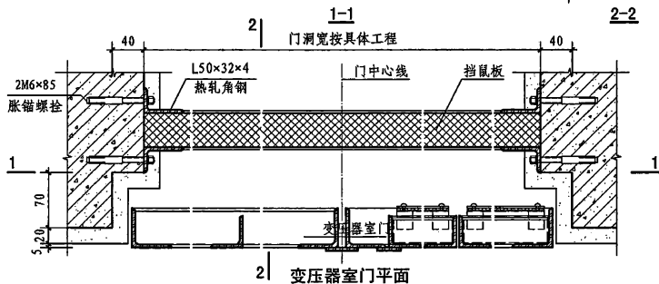
挡鼠板详图
