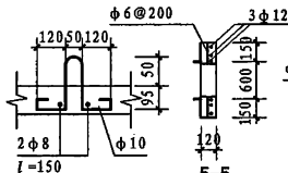
盖板吊环详图
