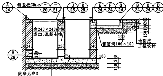
1-1 (砌体沟壁)
