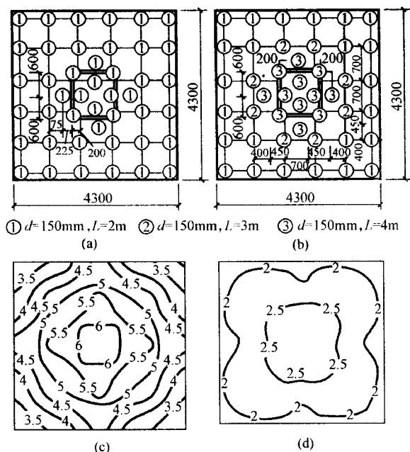
图 6 等桩长与变桩长桩基模型试验 ( P=3250\text{kN} )
