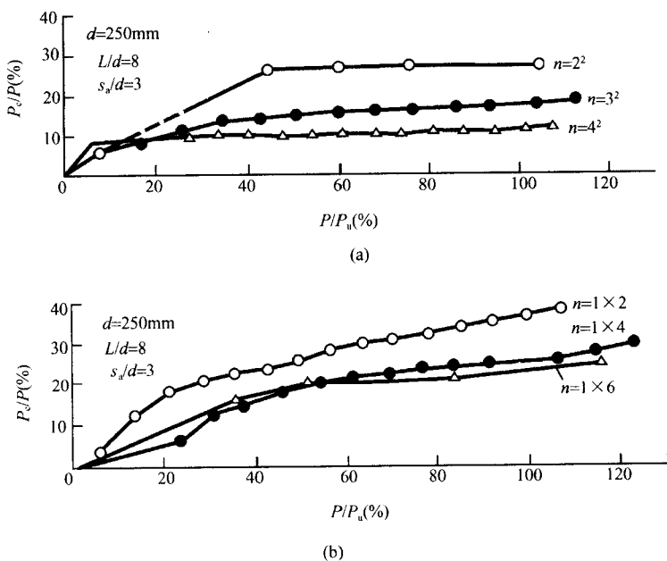
图10 粉土中多排群桩和单排群桩承台分担荷载比 (a) 多排桩; (b) 单排桩
