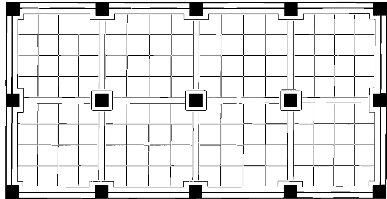
② 水磨石面层分格条平面示意图
