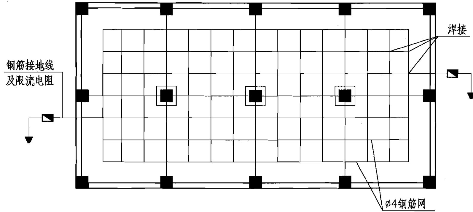
① 方格形导静电接地网
