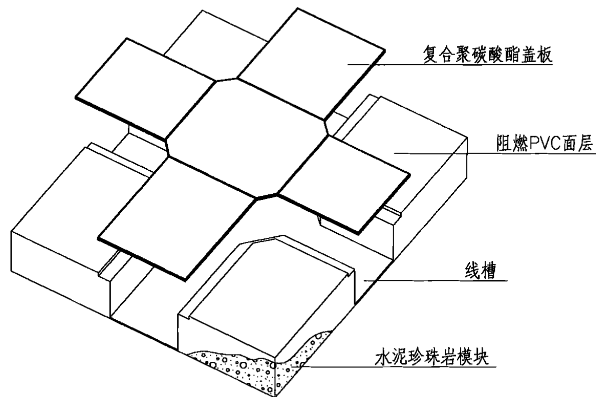
平铺型网络地板结构示意图
