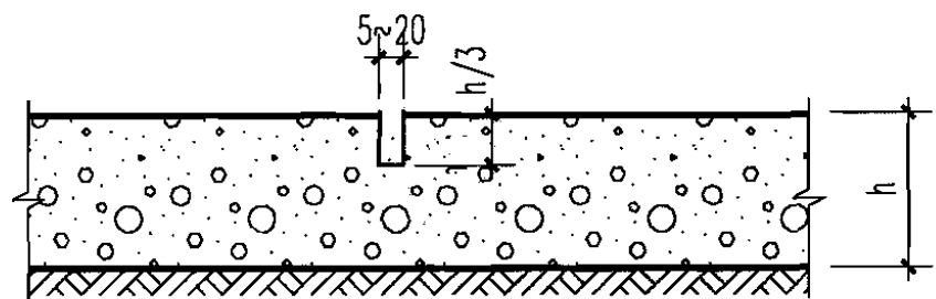
③ 横向缩缝 6 ~ 12m
