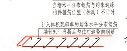
约束边缘暗柱 (一)
