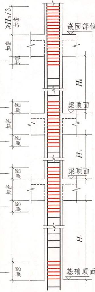
箍筋加密区范围
