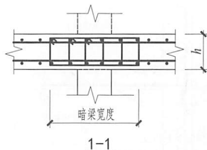
1-1 (暗梁配筋详见设计, 纵向钢筋构造同柱上板带)
