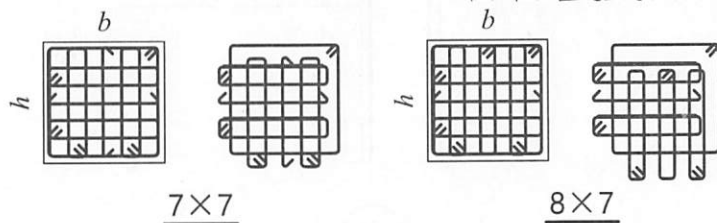
芯柱XZ配筋构造 注：纵筋的连接及根部锚固同框架柱，往上直通至芯柱柱顶标高。
