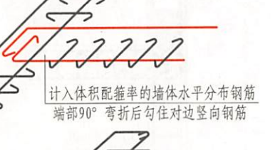
约束边缘翼墙 (一)
