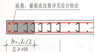
约束边缘暗柱 (二)
