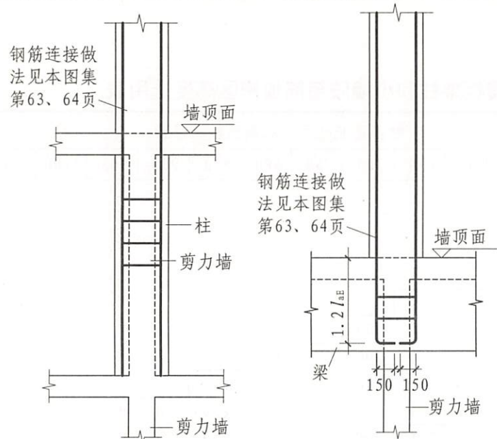
剪力墙上柱QZ纵筋构造
