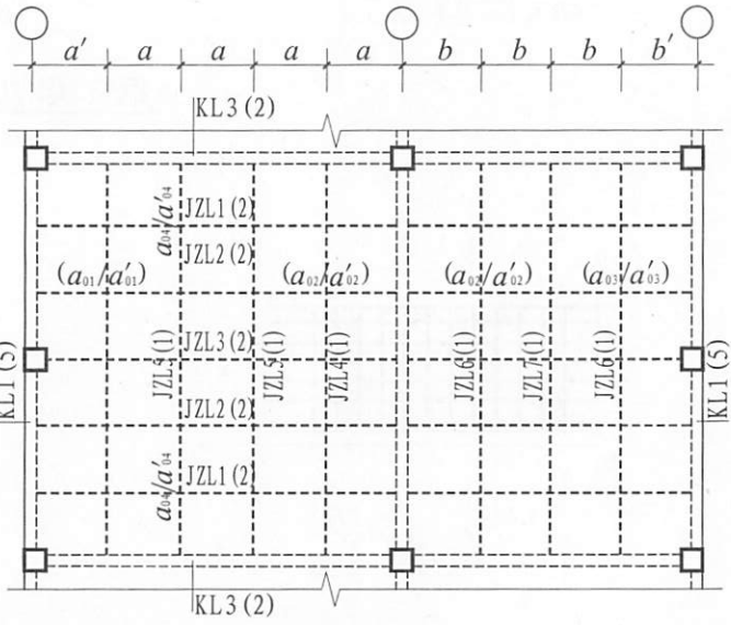
井字梁JZL、JZLg配筋构造
