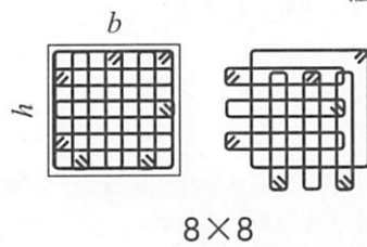
非焊接矩形箍筋复合方式
