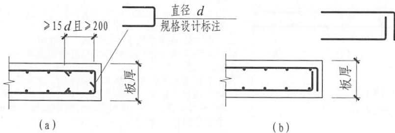
无支承板端部封边构造 (当板厚 \geq 150 时)
