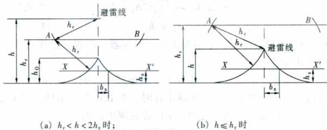
图 B.0.2 单根架空避雷线的保护范围
