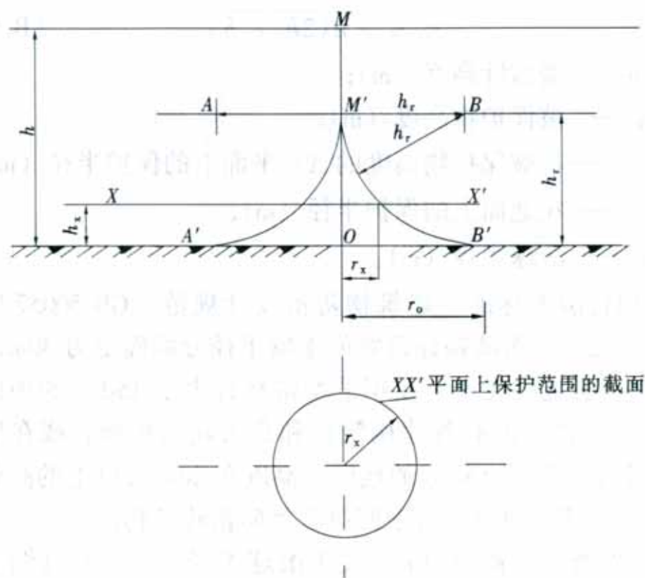
图 B.0.1-2 单支避雷针的保护范围 ( h > h_r )
