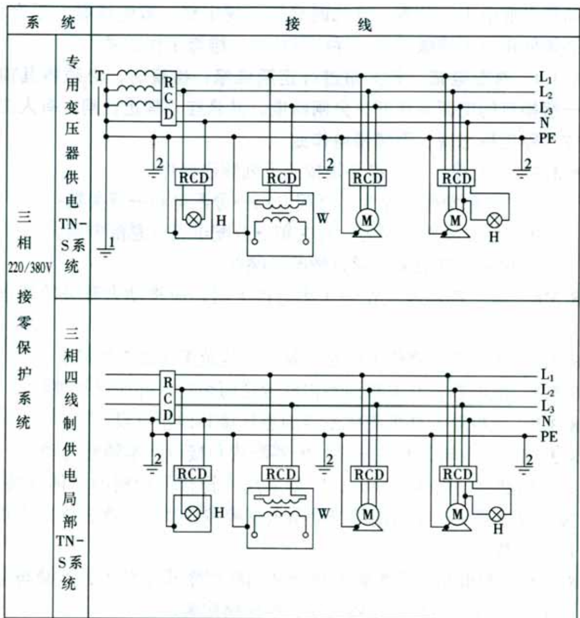
图 8.2.14 漏电保护器使用接线方法示意
