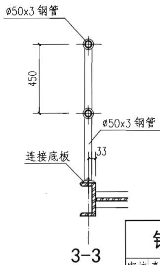
TL18 型
