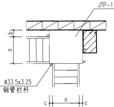
9 靠柱靠墙转角梯间平台
