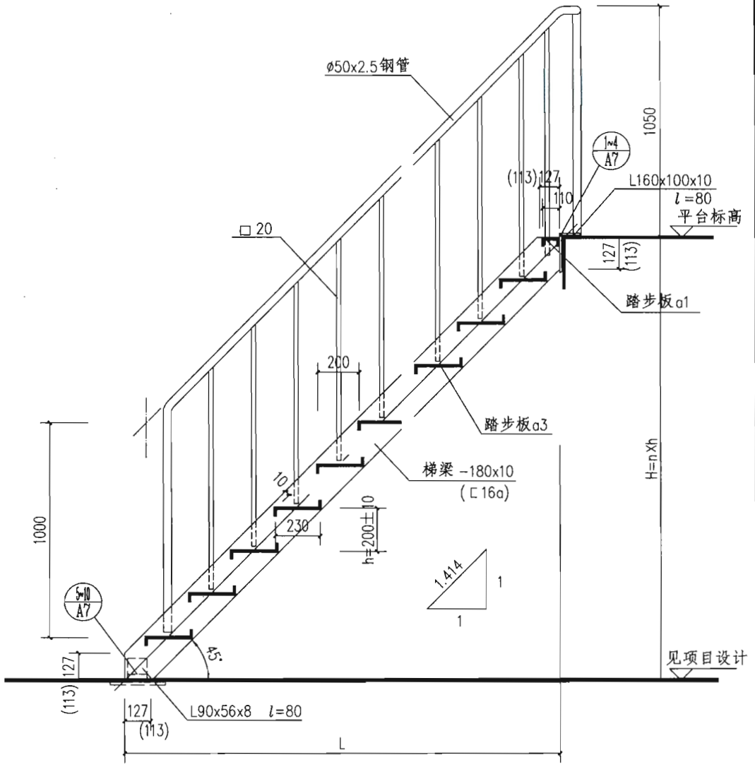
45°钢斜梯 T2A06、T2A08、T2A10 立面、剖面图 T2B06、T2B08、T2B10
