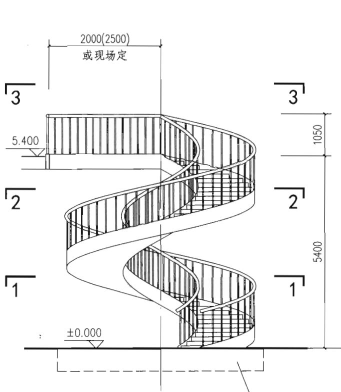
BLTB-5410 立面 (BLTB-5415)
