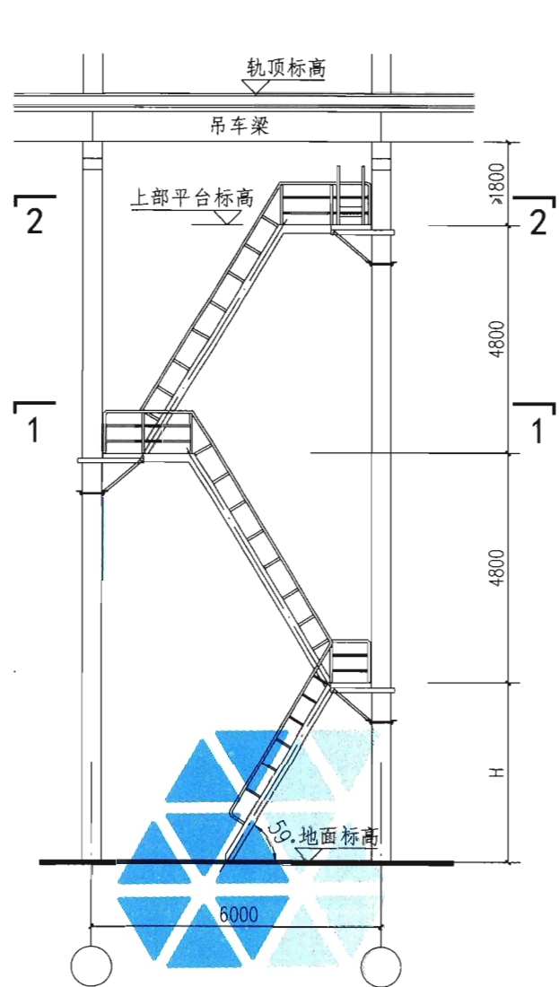
立面
