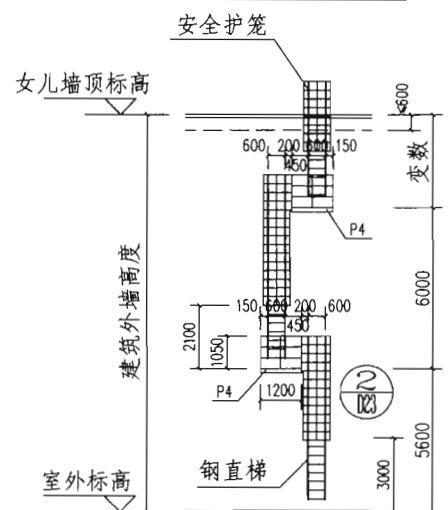
WT3b 立面
