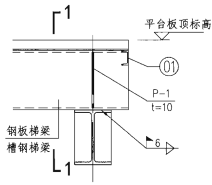
④ 梯梁与平台钢梁 连接节点
