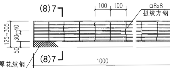
c7 (c8) 型踏步板
