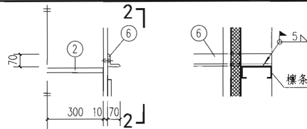
复合板墙上安装
