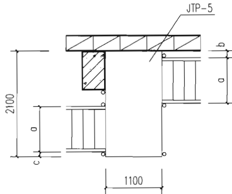
10 靠柱靠墙转角 双跑梯间平台
