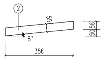
踏步侧板
