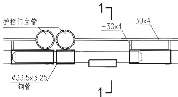
① 门门平面
