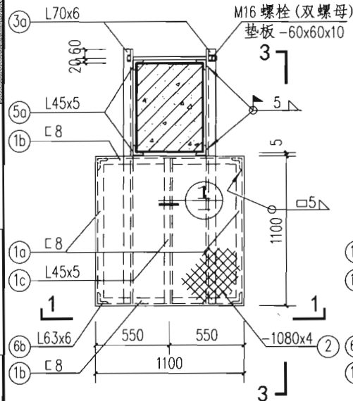
JTP-3平面
