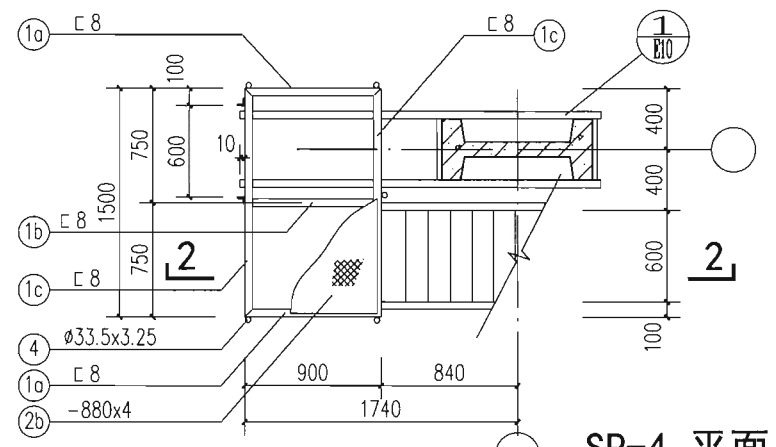
SP-4 平面
