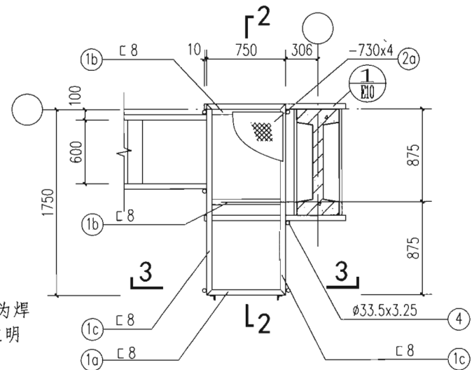
SP-2 平面
