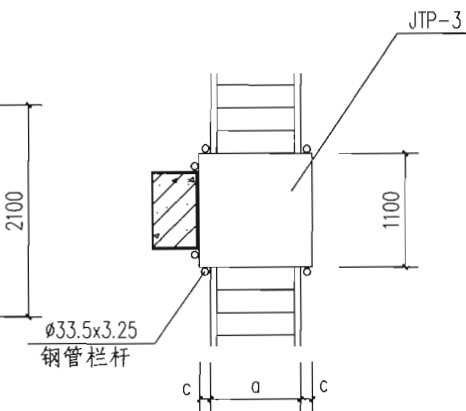
14 靠柱直跑梯间平台
