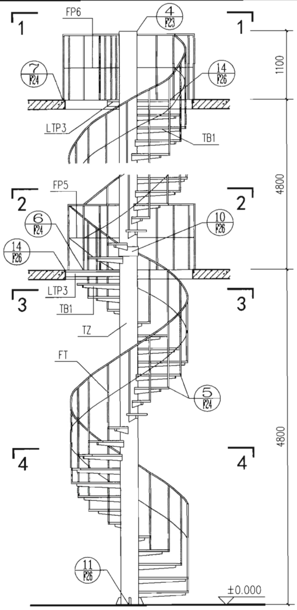
立面
