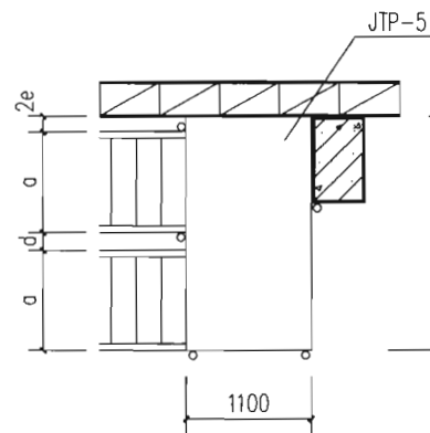
13 靠柱靠墙双跑梯间平台
