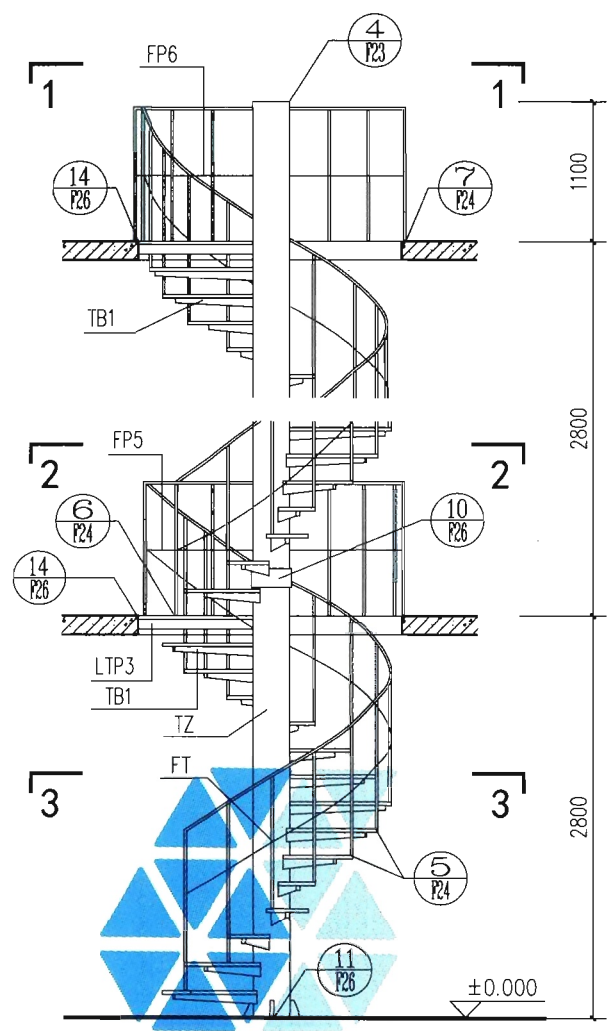
立面
