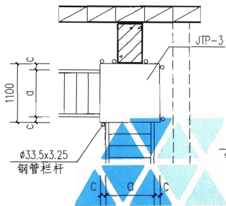
⑤ 靠柱转角梯间平台
