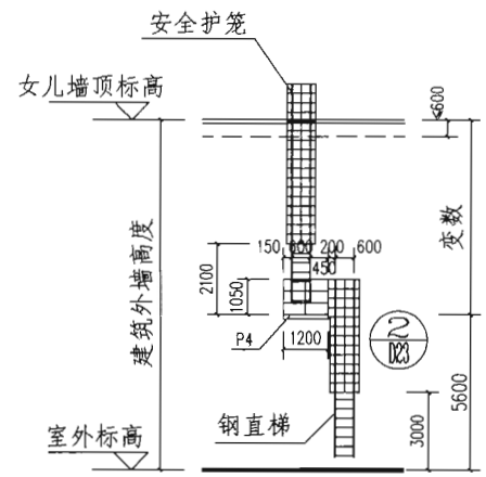
WT3b 立面
