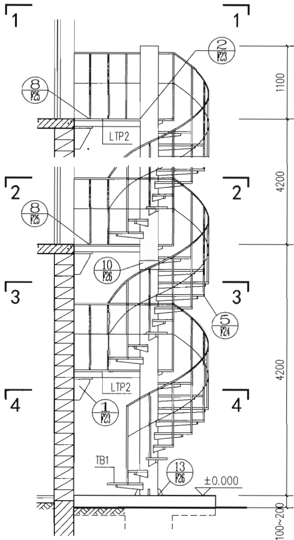
立面
