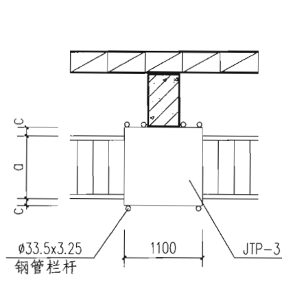
④ 靠柱直跑梯间平台
