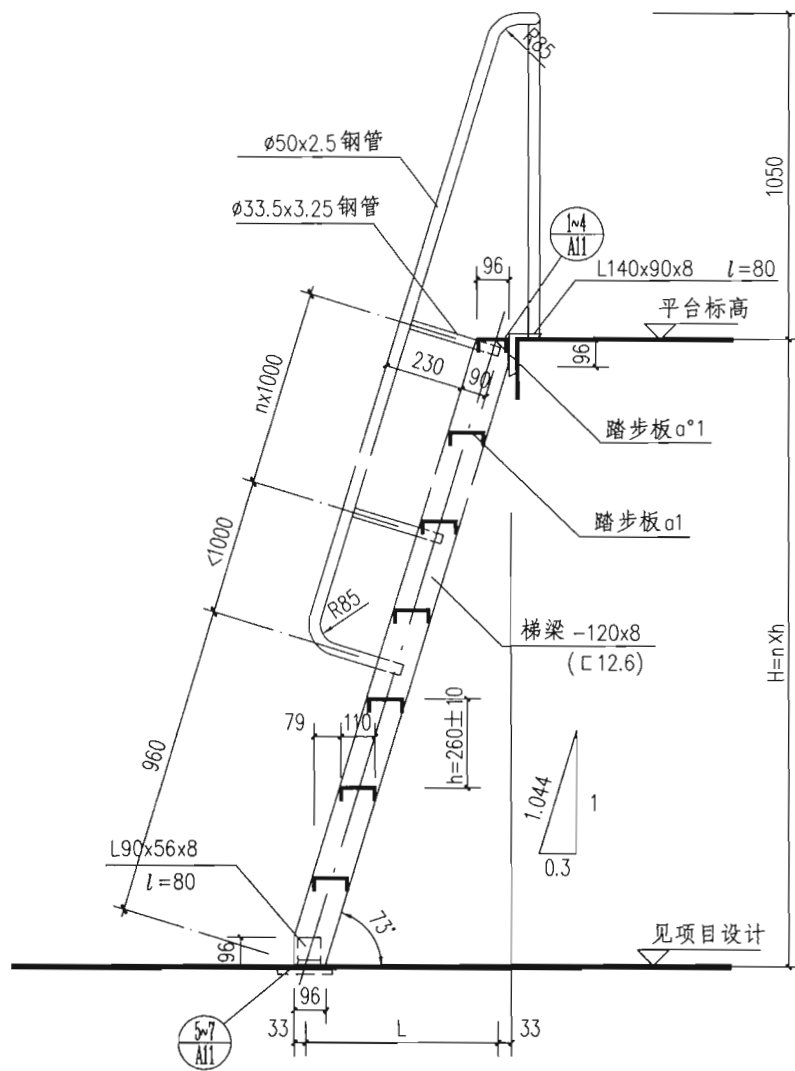
73° 钢斜梯T4A06、T4B06 立面、剖面图
