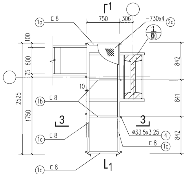
SP-1 平面
