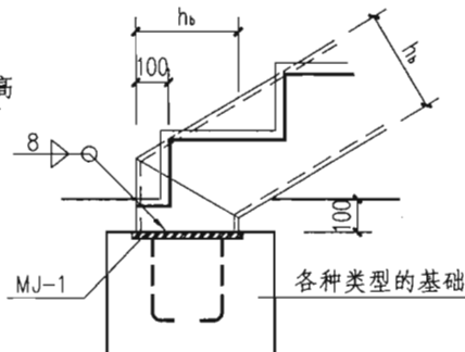
钢梯梁与基础连接构造
