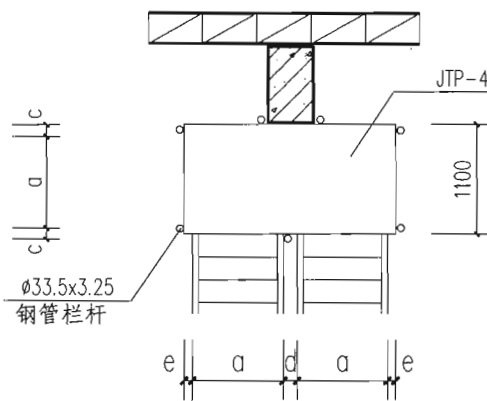
⑦ 靠柱双跑梯间平台
