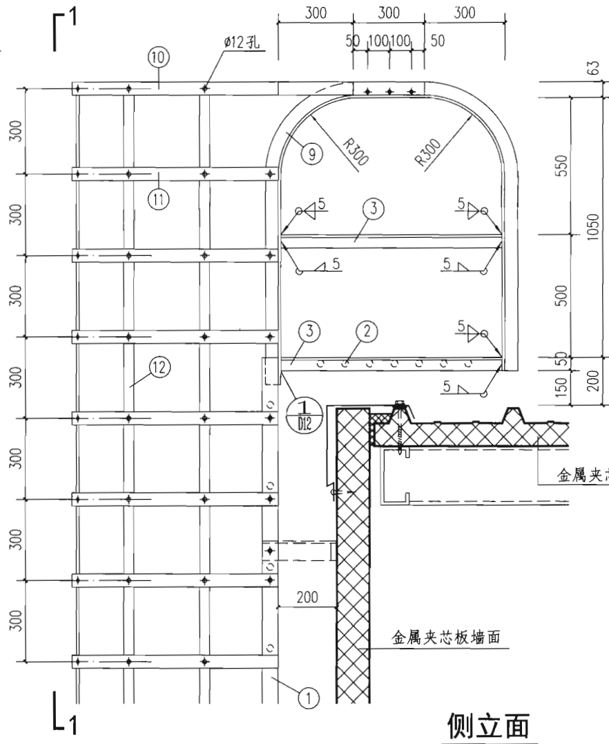
上屋面钢直梯Ab顶段详图(悬挑式)
