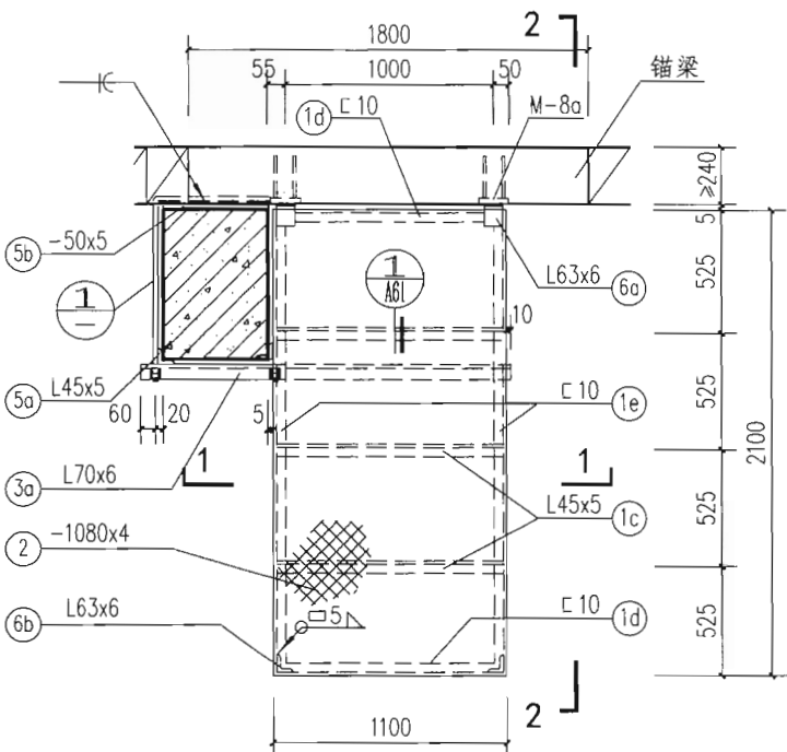
JTP-5平面
