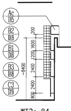
上屋面WT2单段梯钢直梯选用图
