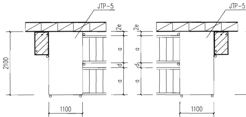
12 靠柱靠墙双跑梯间平台
