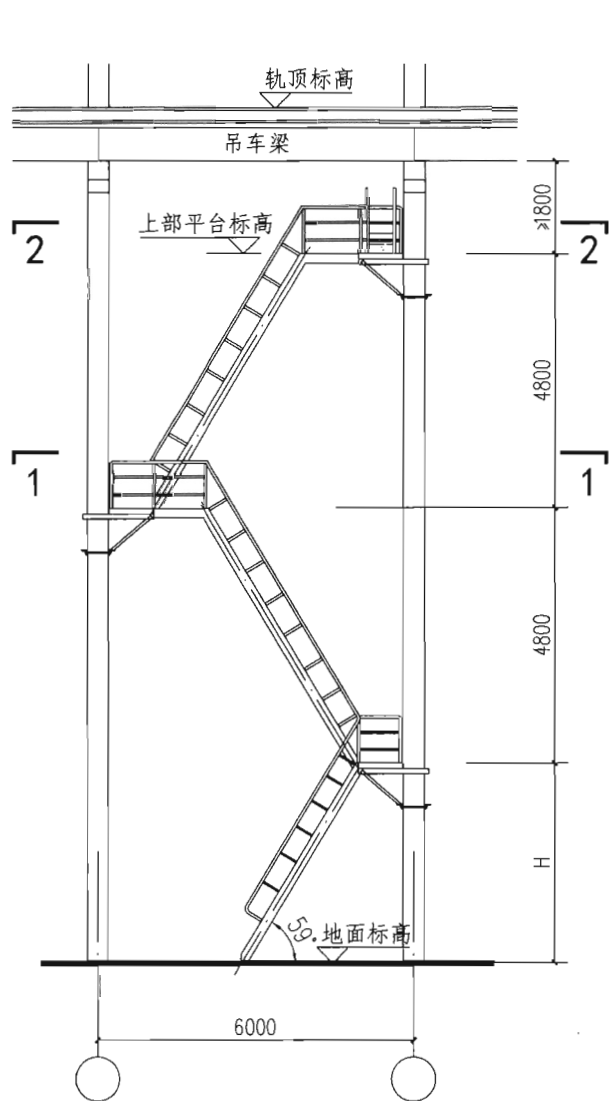
立面
