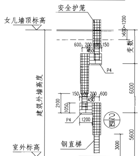
WT3c 立面
