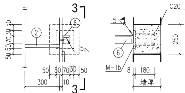
空心砖墙上安装
