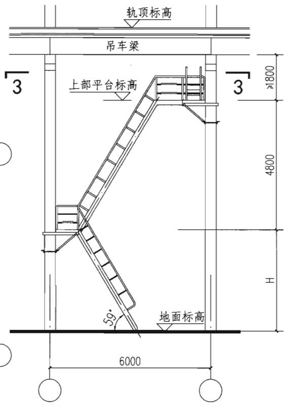
立面
