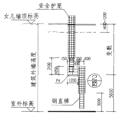
WT3c 立面
