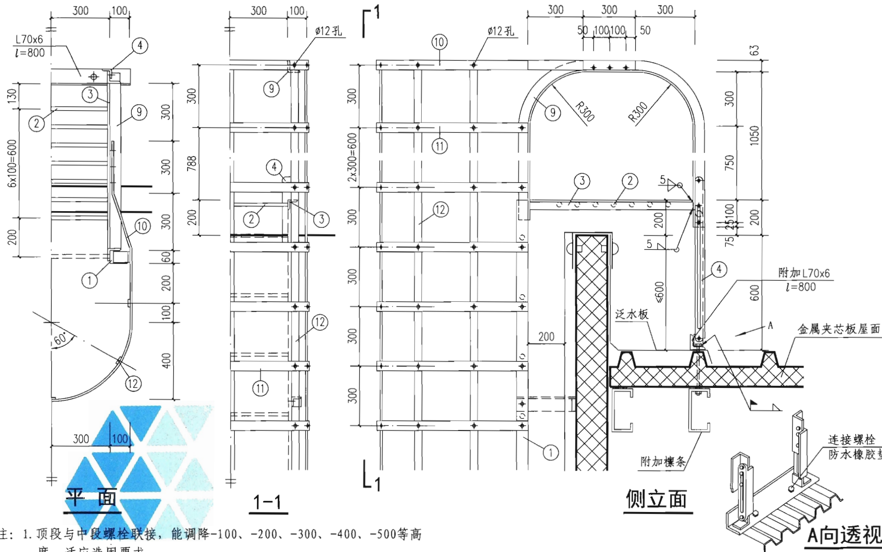
上屋面钢直梯Ab顶段详图(轻型屋面)
