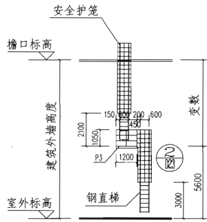
WT3a 立面
