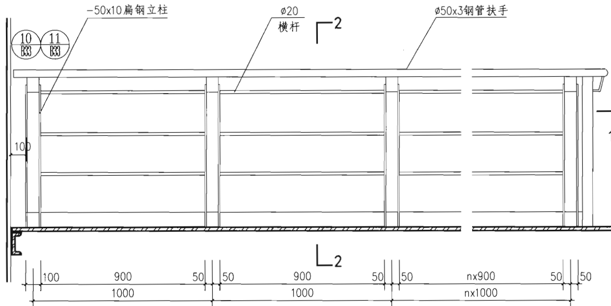
LG14 型立面图
