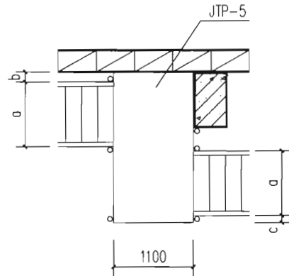
11 靠柱靠墙转角 双跑梯间平台
