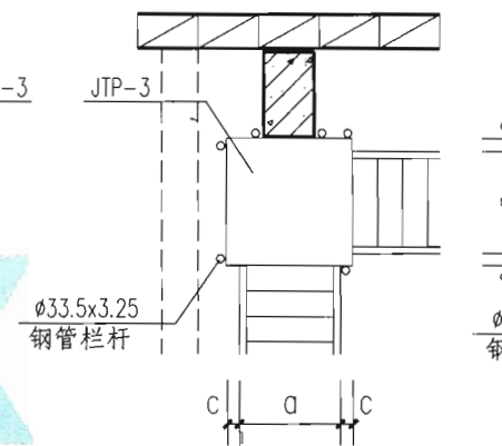
⑥ 靠柱转角梯间平台
