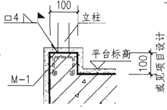
⑨ 混凝土翻边
