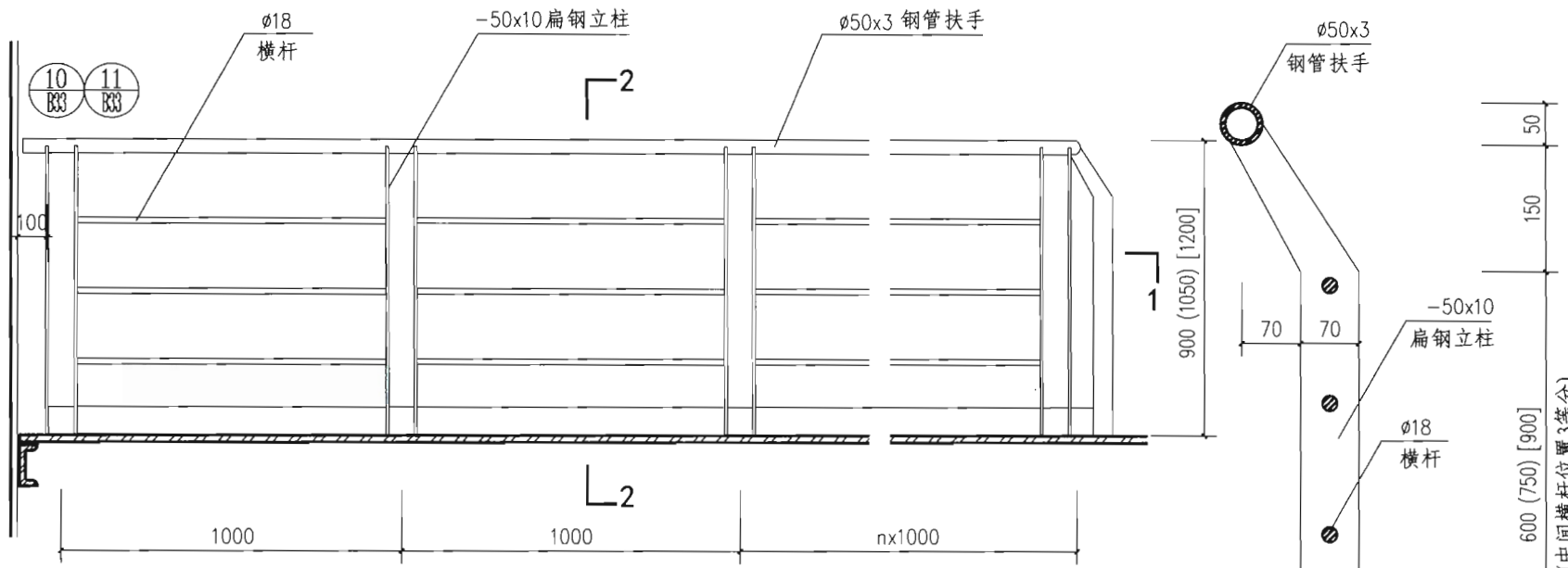
LG13 型立面图
