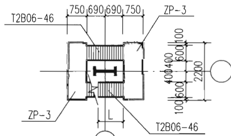
绕柱上吊车钢斜梯简图(73°)
