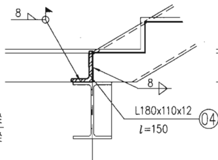
② 梯梁与楼面钢梁 连接节点
