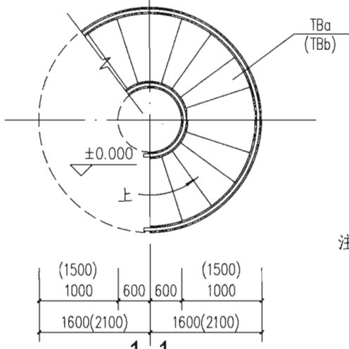
板式钢螺旋梯BLTA-4210、BLTA-4215 简图
