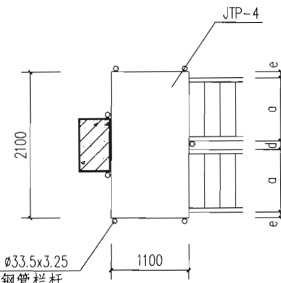
15 靠柱双跑梯间 平台
