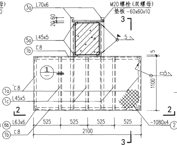
JTP-4平面
