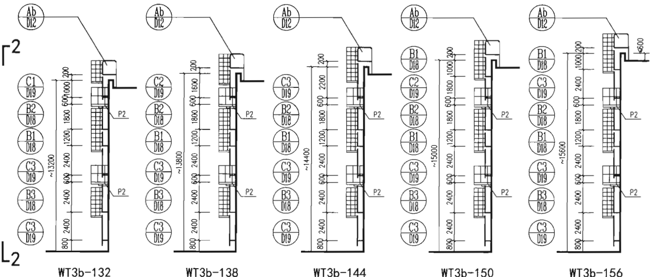
上屋面WT3多段梯下上式钢直梯选用图
