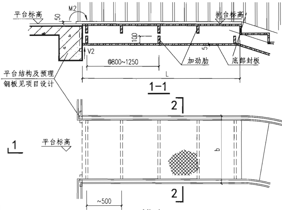
挑台平面
