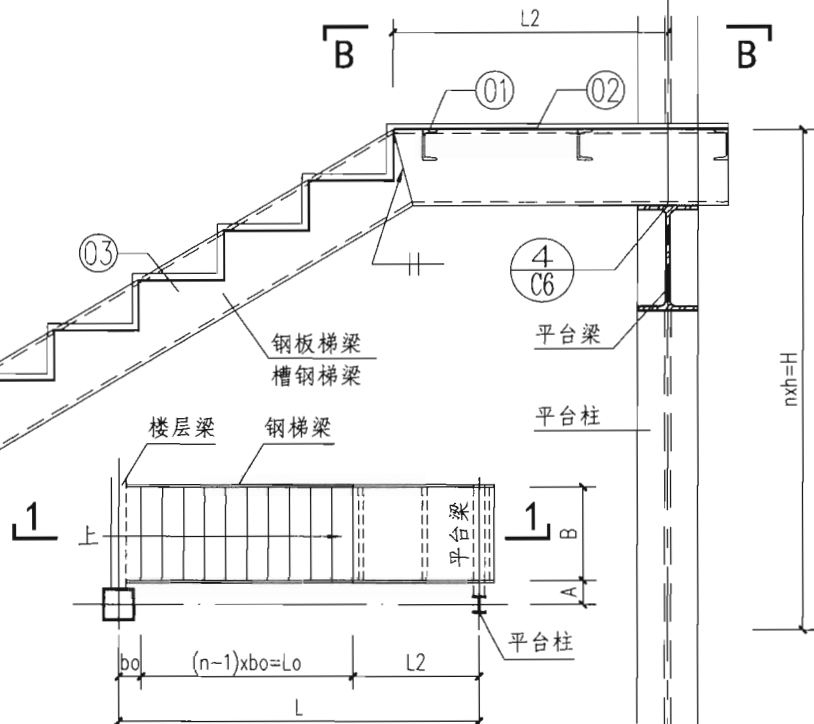
单跑平面布置示意图
